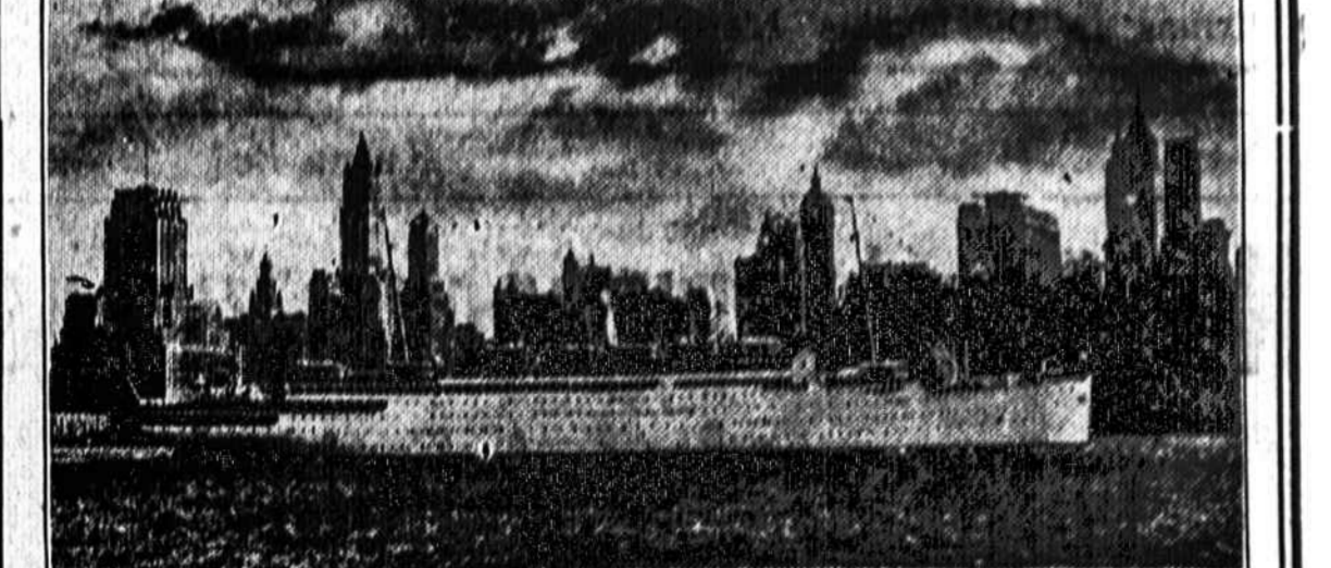
"GRIPSHOLM" Ilgio, 675 pėdų; pločio 74 pėdų; 18,000 reg. tonų tonazas; įtalpos 23,000 tonų.
