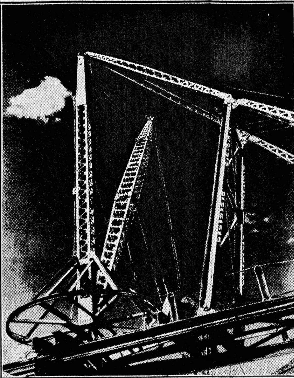
STATO TVENKINĮ. — Vaizdas prie Columbia upės, Washington, kur federalės valdžios lėšomis yra statomas Grand Coulee tvenkinys. Paveikslas parodo milžinišką kraną, kuriuo pilama cementas į tvenkinio sieną. Kėnas vienu sykiu pakelia keturis kubinius jardus cemento.
