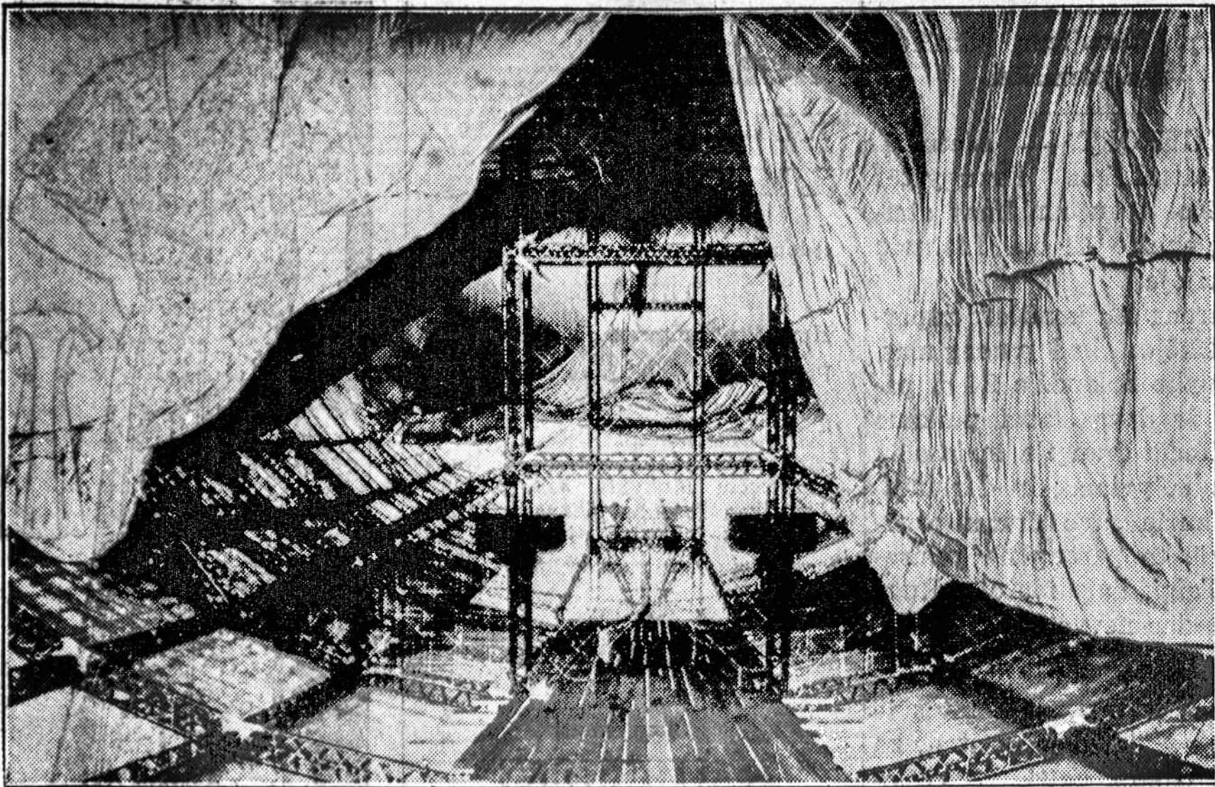
ŽUVUSIO VOKIEČIŲ DIRIZABLIO "HINDENBURGO" VIDUS. PAVEIKSLAS parodo jo konstrukciją. Iš šalies nusidriekę maišai, kurie buvo užpildyti sprogstančiomis vandenilio (hydrogen) dujomis.
