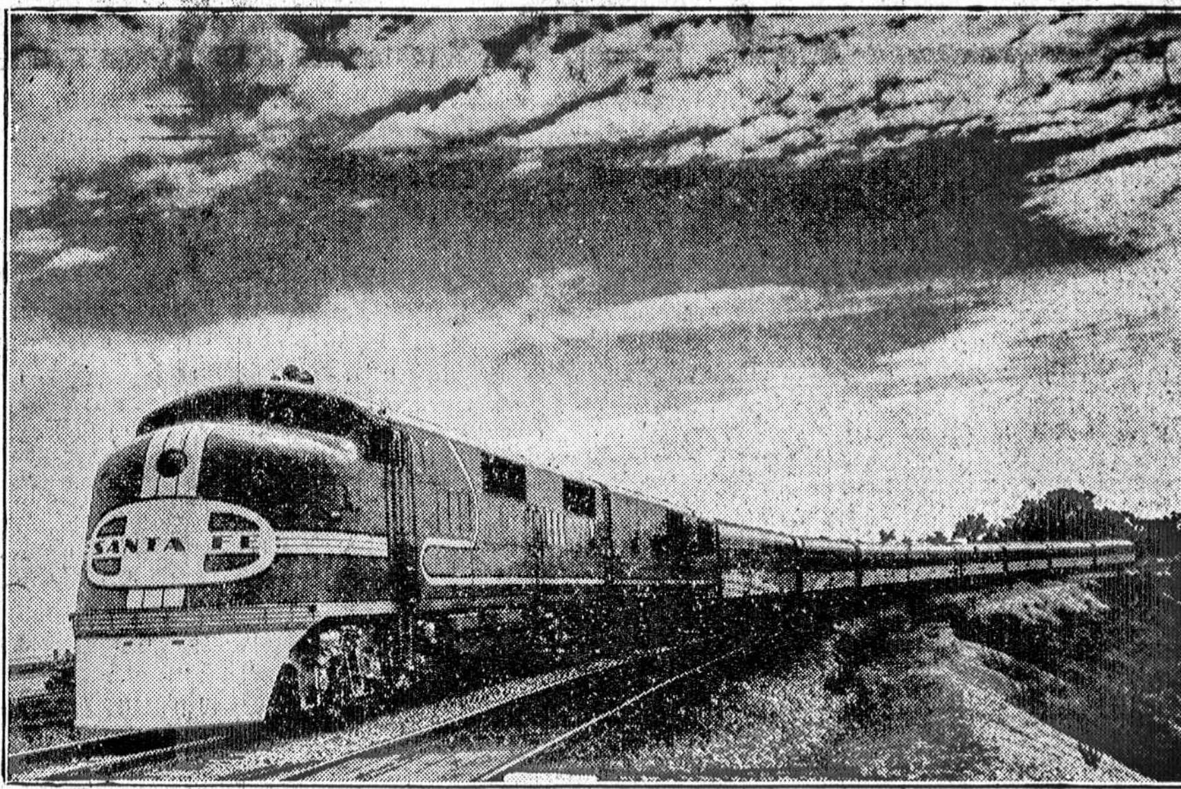
VĖLIAUSIA NAUJIENYBĖ ANT BĖGIŲ — "The Super Chief" liuksusinis Santa Fe gelžkelio traukinys, kuris vakar buvo bandomas Chicagoje. Sakoma, kad jisai padarys kelionę iš Chicagos į Los Angeles į 39 valandas, 40 minučių. Dieselinis motoras išvysto 3,600 arklių jėgą.
