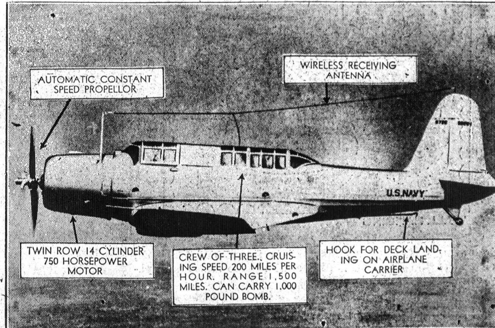
NAUJI SPARNAI LAIVYNUI — Paveikslas parodo modelį 54 bombanešių lėktuvų, kuriuos nupirko J. V. oro laivynas. Lėktuvas yra daug greitesnis ir gali daugiau pakelti negu jo pirmtakui. Acme Photo
