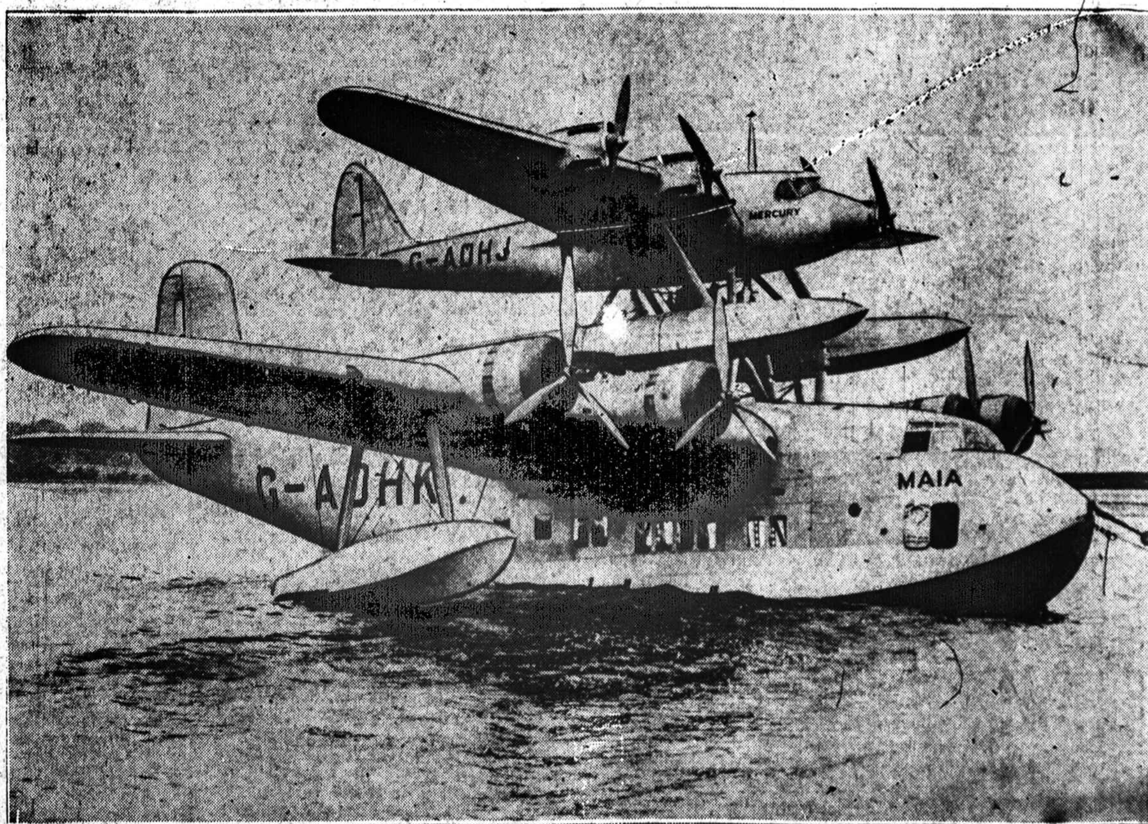
SUDĖTINIS LĖKTUVAS. — Anglijoje tapo pastatytas sudėtinis lėktuvas "Pick-a-Back", kuris ištikrųjų susideda iš dviejų lėktuvų, vienas ant kito. Tokis lėktuvas yra skiriamas skridimams per Atlantiką ir manoma, kad tokių lėktuvų įstengs paimti didesnę krovinių prekių ir pasażierių.
