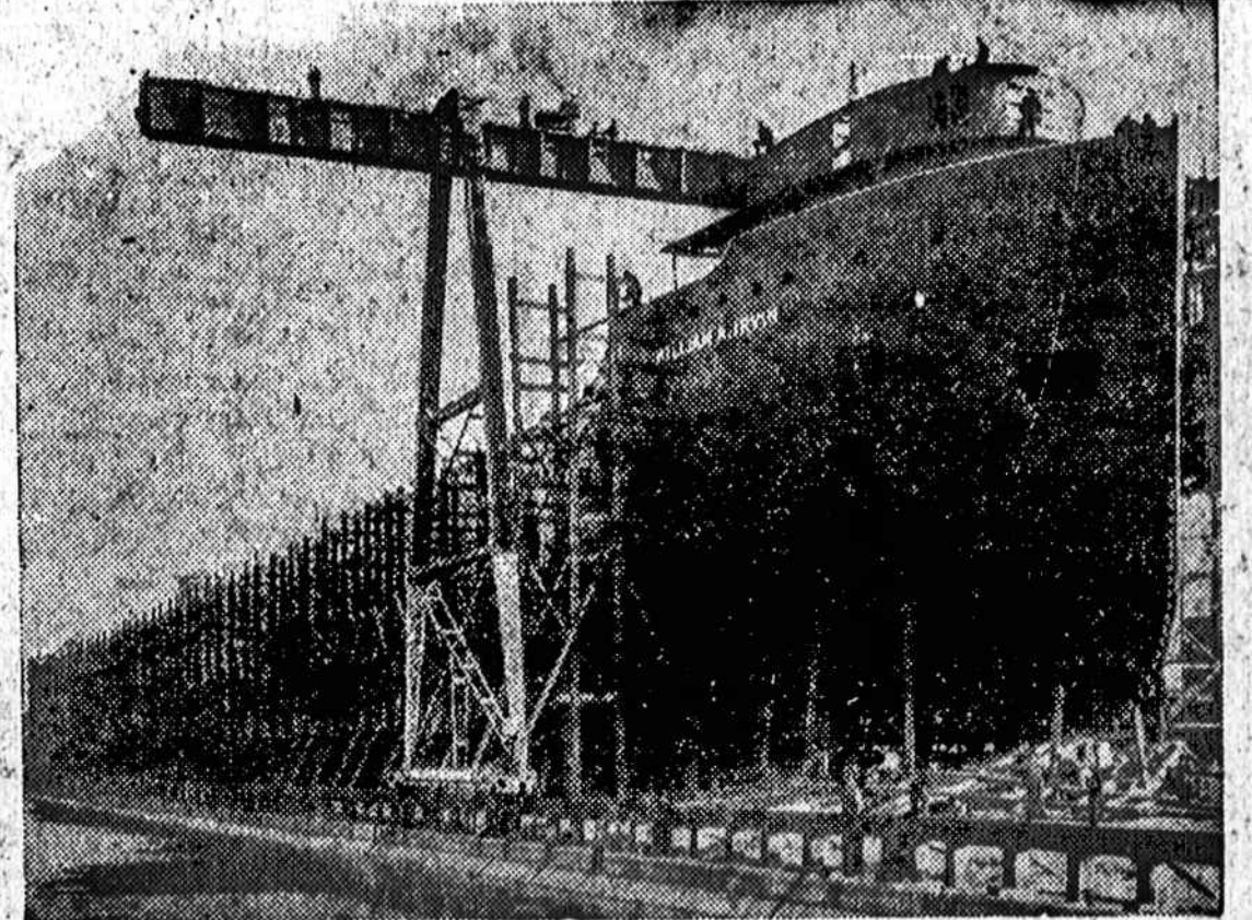
GELEZIES RUDOS LAIVAS. — Baigiamas statyti United States Steel Corp. geležies ruda gaminti laivas William A. Irvin, 610 pėdų. Jis statomas Lorain, O. ir bus pirmas per septynis metus pastatytas naujas laivas dėl Didžiųjų Ežerų.
