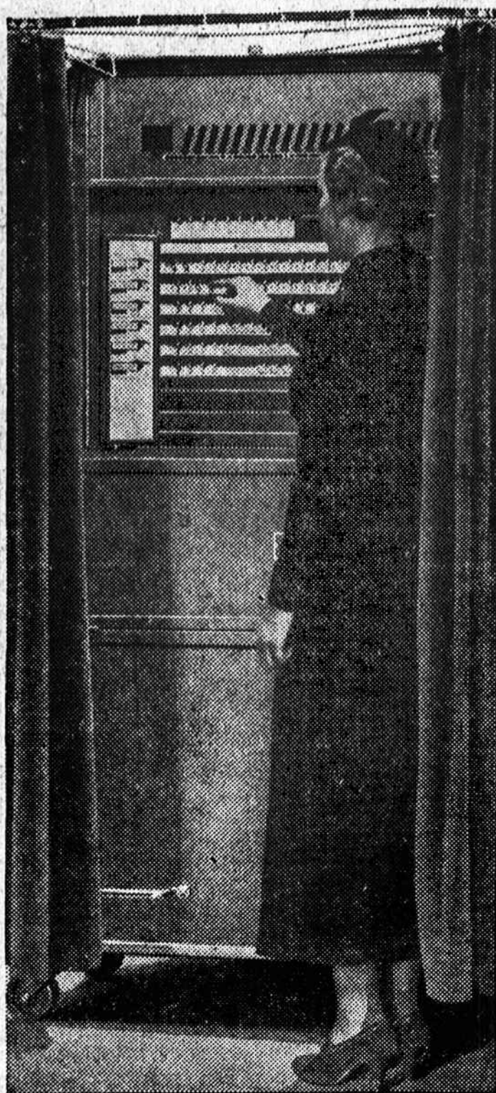
Paveikslas parodo kaip Balsavimo Mašina išrodo ir kaip operuojama
