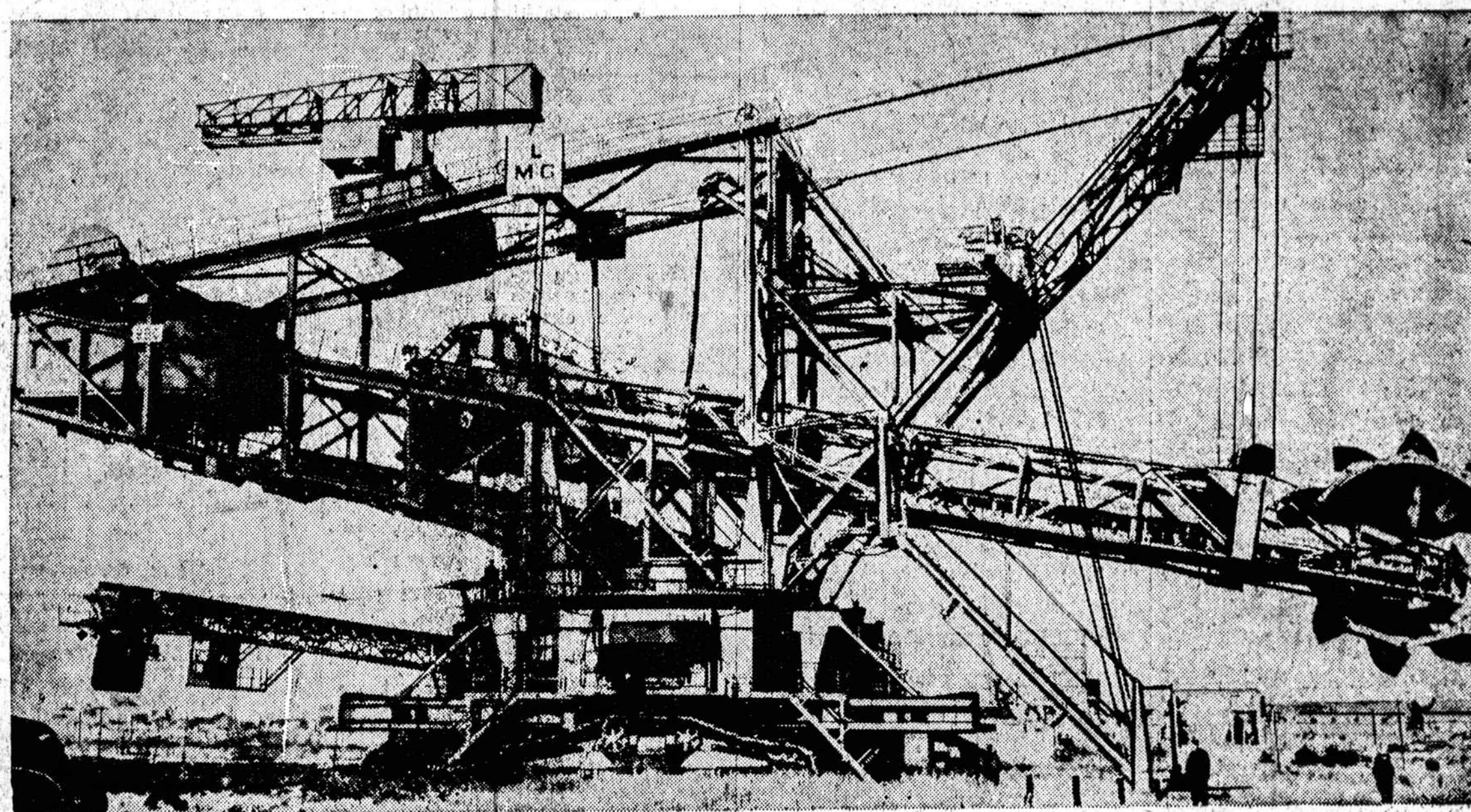
DIDŽIAUSIAS SĖMTUVAS PASAULYJE. — Mlžiniškas, didžiausias pasaulyje sėmtuvas, įrengtas Bitterfelder Bezirk kasyklose, Vokietijoje. Mašina turi 25,000 kubinius metrus įtalpos.
