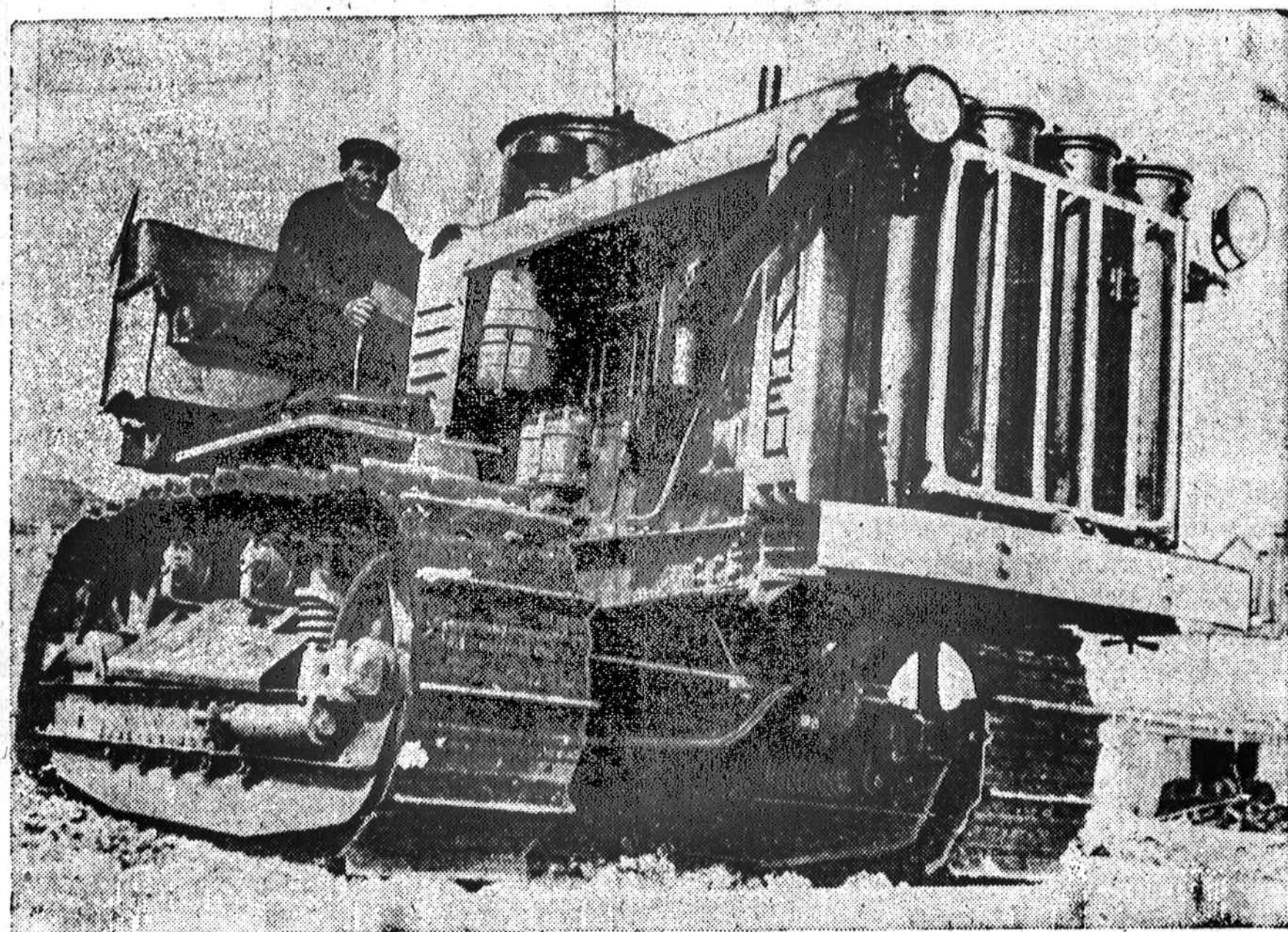
Pirmas rusų traktorius, kurs važiuoja savo padaromu gasu. Mašinos motoras yra 75 arklių pajėgos. Generuoja didelio degimo gasą iš pigios medžiagos.
