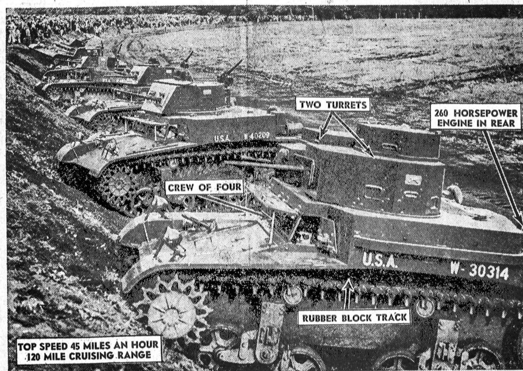
Naujausio modelio amerikoniškos tankos, kurios buvo rodomos armijos oficerams ir industrialistams Rock Island arsenale. Priešakinė tanka yra mažesnio modelio ir gali važiuoti 45 mylių į valandą greitumu.
