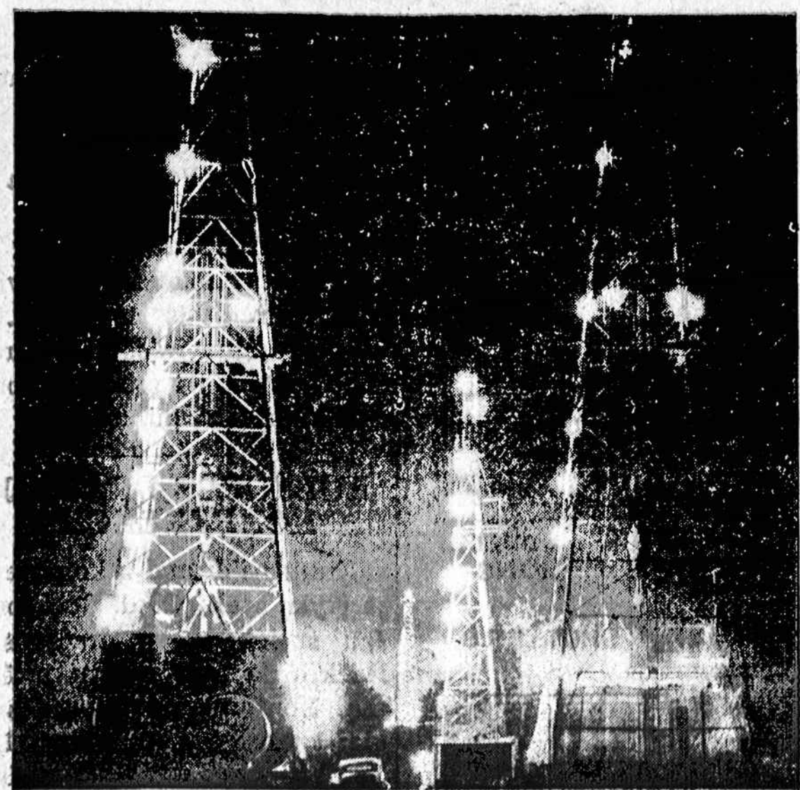
Salem naftos laukas Marion kaunteje nakties metu. Illinois naftos (mineralinio aliejaus) produkcijos atžvilgiu užėmė jau ketvirtą vietą tarpe valstijų. Iš Salem Pool gaunama apie 55 nuos. visos Illinois naftos. 1939 metais buvo priskaitoma 1,577 aliejaus šuliniai. Per dieną naftos gaunama iki 300,000 bačų.
