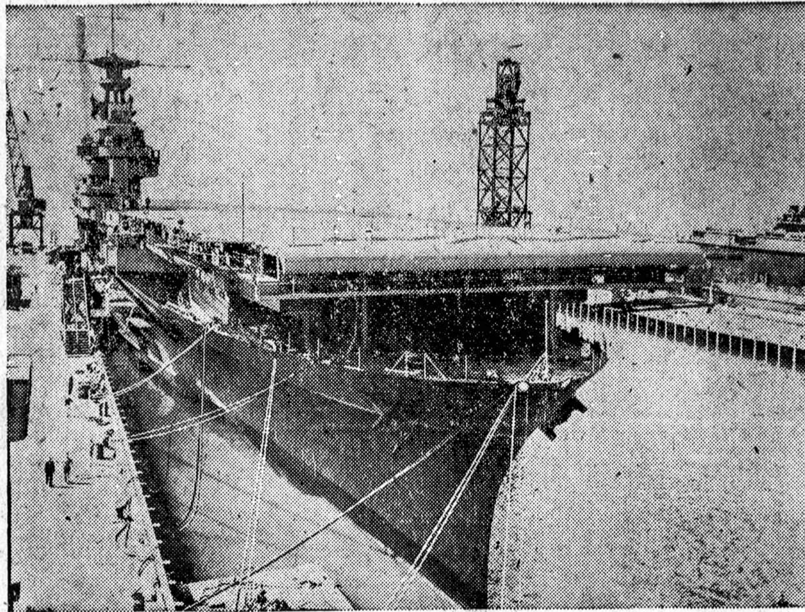
U. S. S. Hornet, naujasis 20,000 tonų lėktuvnešis, vakar perduotas J. V. Laivynui. Laivas gali išvystyti 30 mazgų per valandą greitį.
