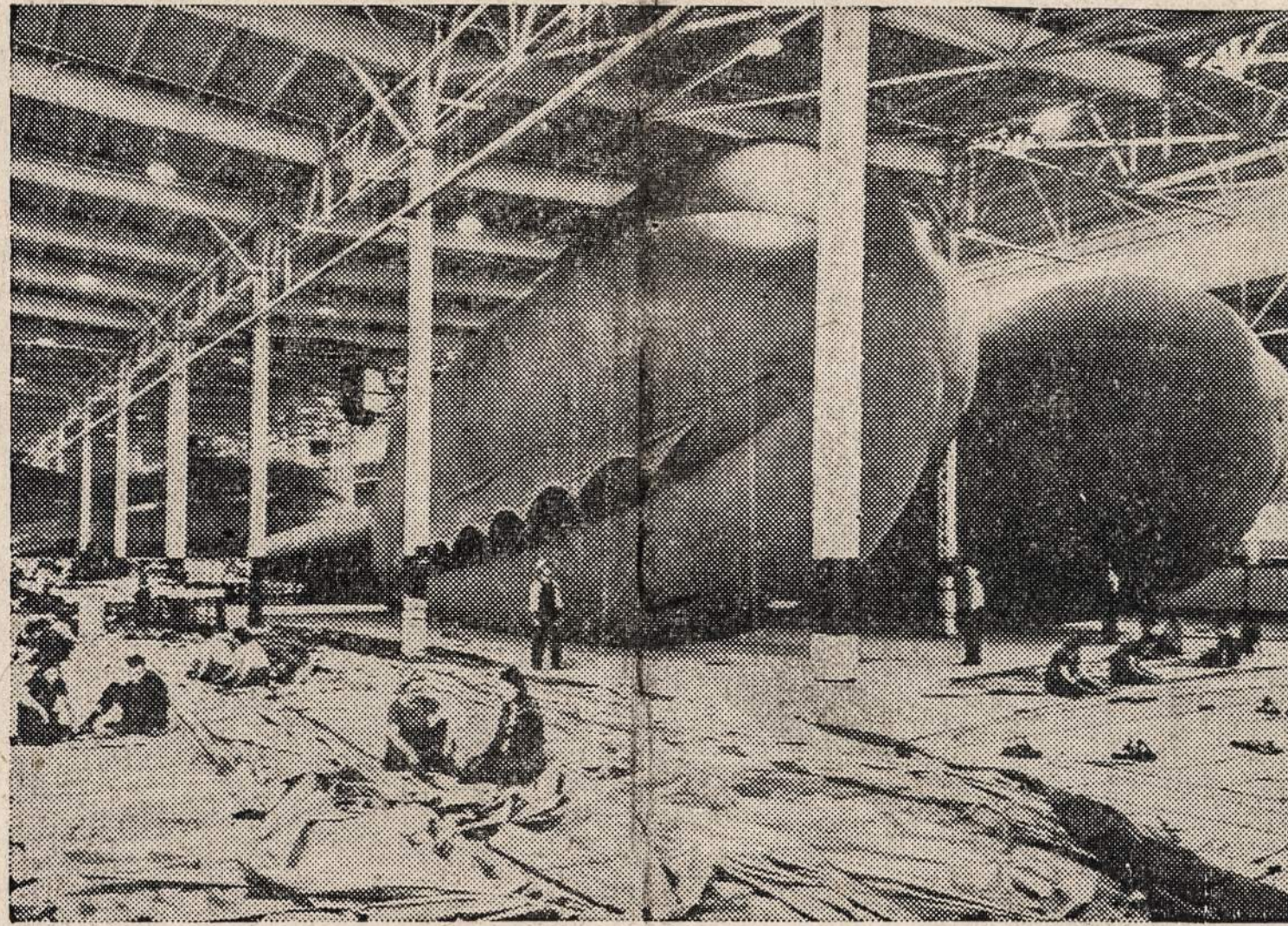
Akrone, Ohio, Firestone Tire and Rubber Co. inžinieriai daro paskutinius bandymus su naujai pagamintais balionais, kurie bus naudojami balionų užtvarams apsigynimui nuo lėktuvų.
