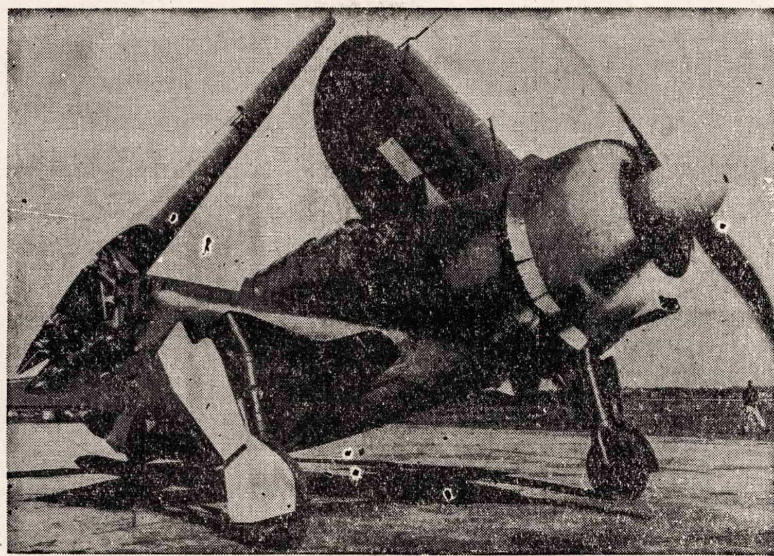
Naujas Curtiss Helldiver nardomas bombonešis, kuris yra SB20. Bombonešis gali operuoti iš sausumos bazių bei lėktuvnešių.
