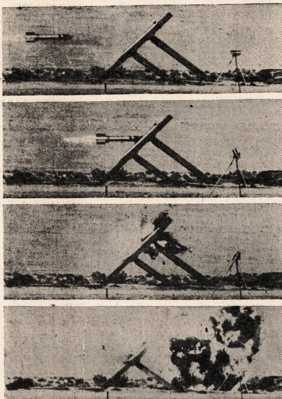
INYOKERN, Calif. — Laivyno pareigūnai demonstruoja naują raketą, kuri vadinama "Tiny-Tim". Raketa permuša storą plieno taikinį ir eksploduoja.
