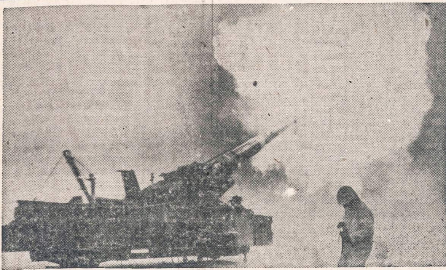
KOMBINUOTAS PABŪKLAS. — Armija nuėmė šydą nuo 85 tonų kilnojamo 230 mm. artilerijos pabūklo, galinčio šaudyti normaliais ir atominiiais sviediniais. Pabūklas yra 4 kartus taiklesnis už bet kurį ligi šiol naudotą artilerijos pabūklą ir gali puikiai remti sausumos kariuomenę bet kokiose oro sąlygose, dieną ir naktį. Jis gali būti perkeliamas iš vienos vietos į kitą, laukais ar keliais, apie 35 mylių per valandą greičiu ir tinka išsikėlimui iš jūros.
