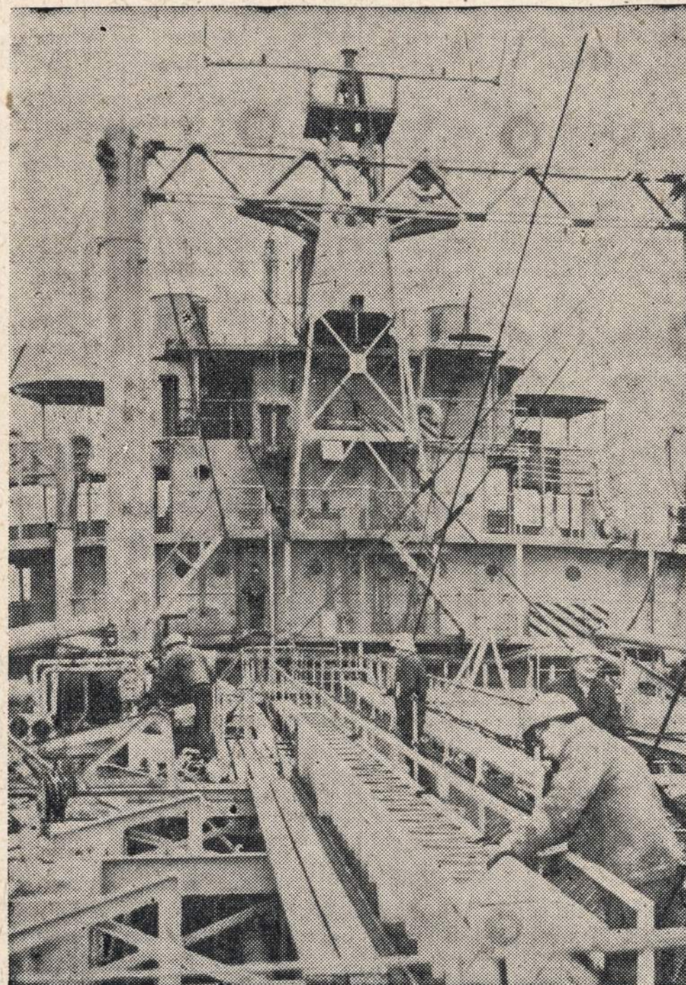
Laivas USS Kankakee yra atremontuojamas Philadelphia dirbtuvėse. Jis bus panaudotas žibalo transportavimui Vakarų Europai.
