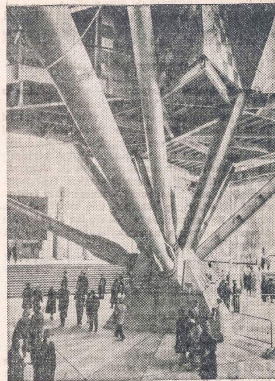
Nepaprastos struktūros prancūzų paviljonas pasaulinėje parodoje, kuri vyksta Bruselyje, Belgijoje. Paviljonas yra labai tvirtas ir labai lengvai išgriaunamas. Jį suprojektavo architektas Guillaume Gillet.
