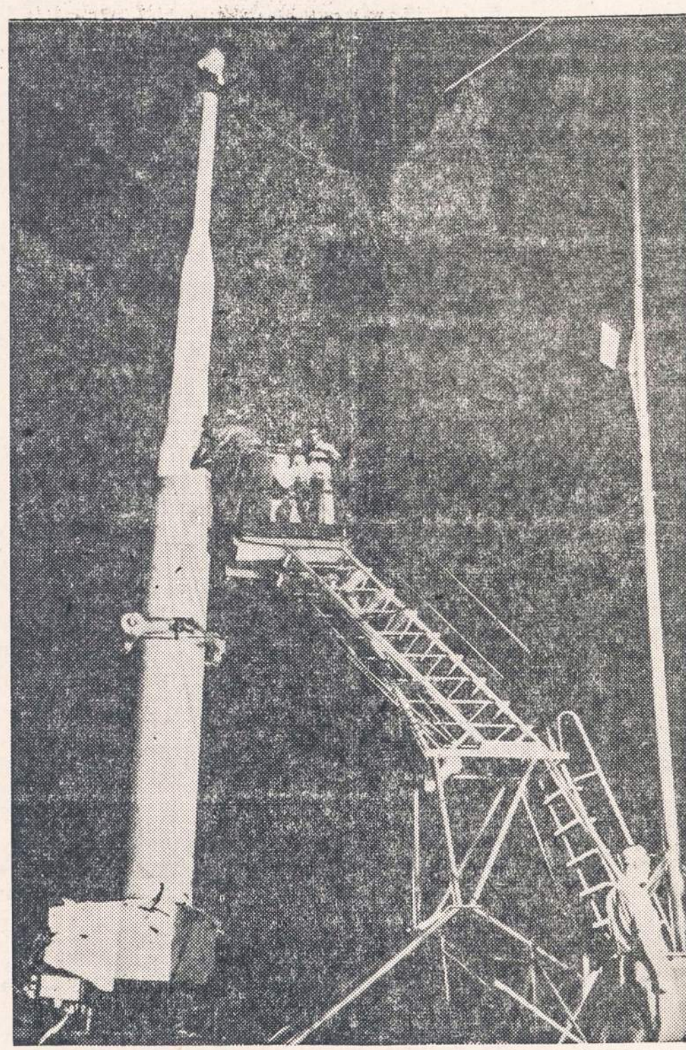
Keturiasdešimt pėdų aukštumo Lockheed X-17 balistinė raketa yra patikrinama prieš paleidimą iš Cape Canaveral (Florida).
