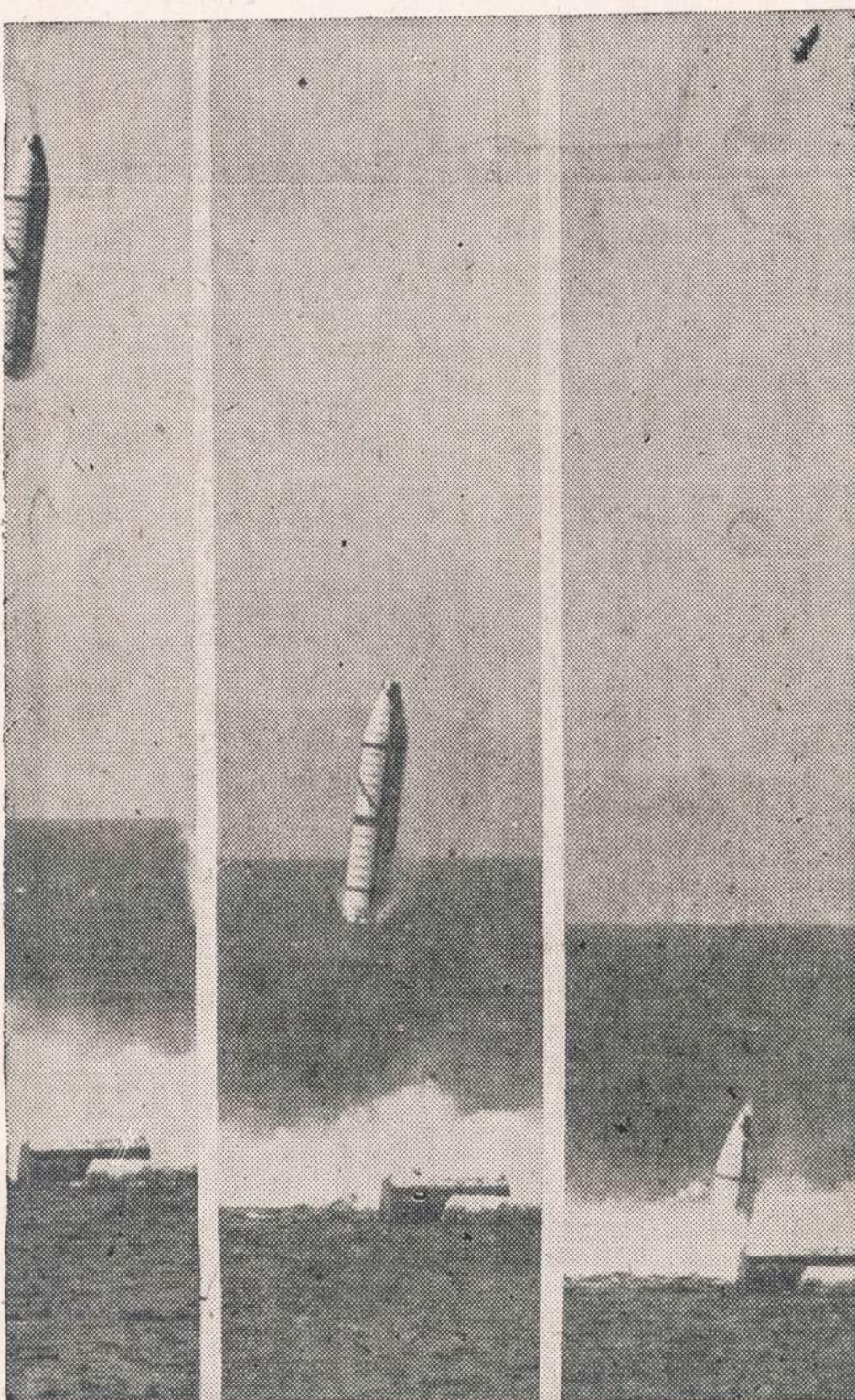
Polaris sviedinys, iššautas iš po vandens, krinta atgal. Povandeninis tinklas nukritusį užtaisą vėl sužvejoja. Bandymas buvo padarytas visai taip, kaip jis bus daromas, sviedinį išsaulant iš povand. laivo.
