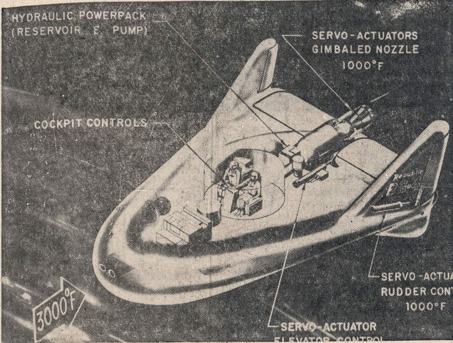
Republic Aviation Corp. suplanuotas erdvio laivo pavyzdys, rodo kritiškai aukštą temperatūrą laivui iš erdvio grįžtant atgal į žemės atmosferą. Republic, pradėjusi 35 milijonų dolerių projektą "karštieji barjerai" ir kitoms erdvio problemoms spręsti, baigianti išrasti metalo liejinį, kuris galės atlaikyti 1,000 laipsnių karščio.
