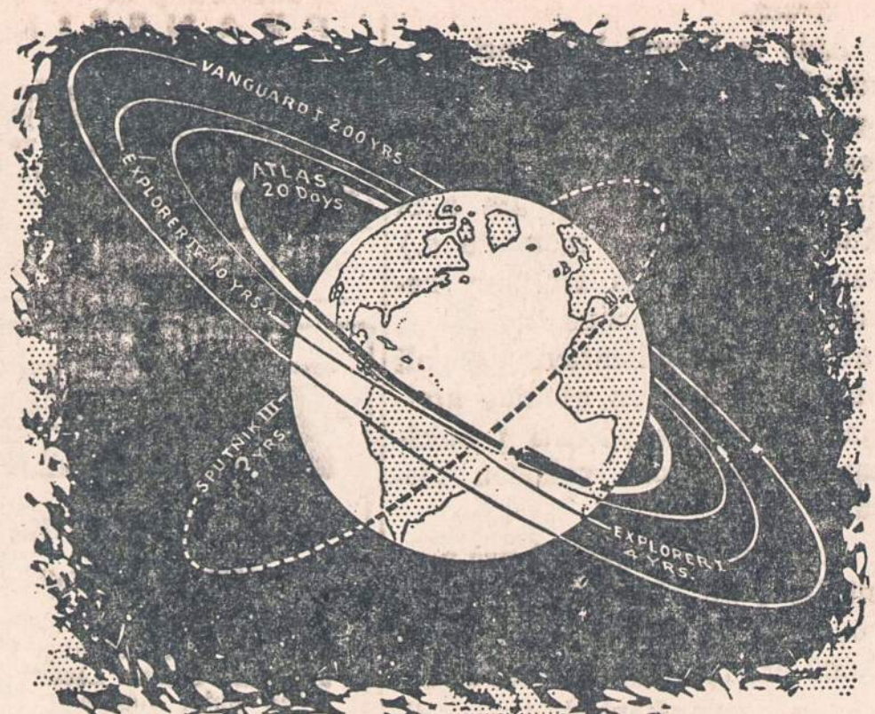
Šis piešinys parodo satelitus, kurie sukasi aplink žemę. Pažymima ir laikas, kaip ilgai jie dar suksis. Vienas satelitas yra rusų, o kieturi Jungtinių Amerikos Valstybių. Vėliausias ir didžiausias Amerikos satelitas Atlas buvo paleistas prieš keletą dienų.
