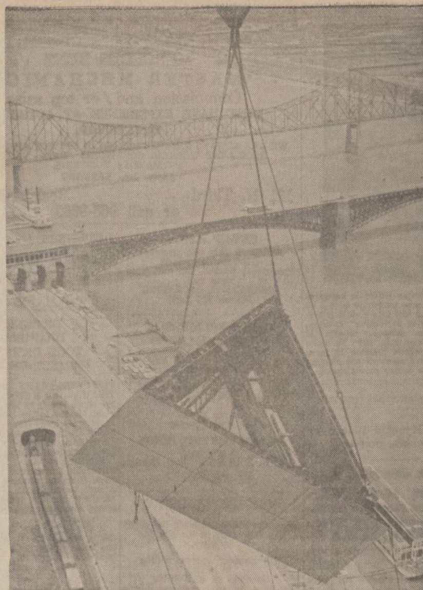
Praeitais metais St. Louis mieste buvo pastatyti Vartai ir Vakarai. Tai milžiniška nerūdijamo plieno arka, suplanuota architekto Eero Saarinen ir iškilanti virš visų tiltų ir pastatų. Paveiksle inžinieriai kelia į arkos viršūnę paskutinę plieno pleiską, kuri sujungė abu arkos sparnus.
