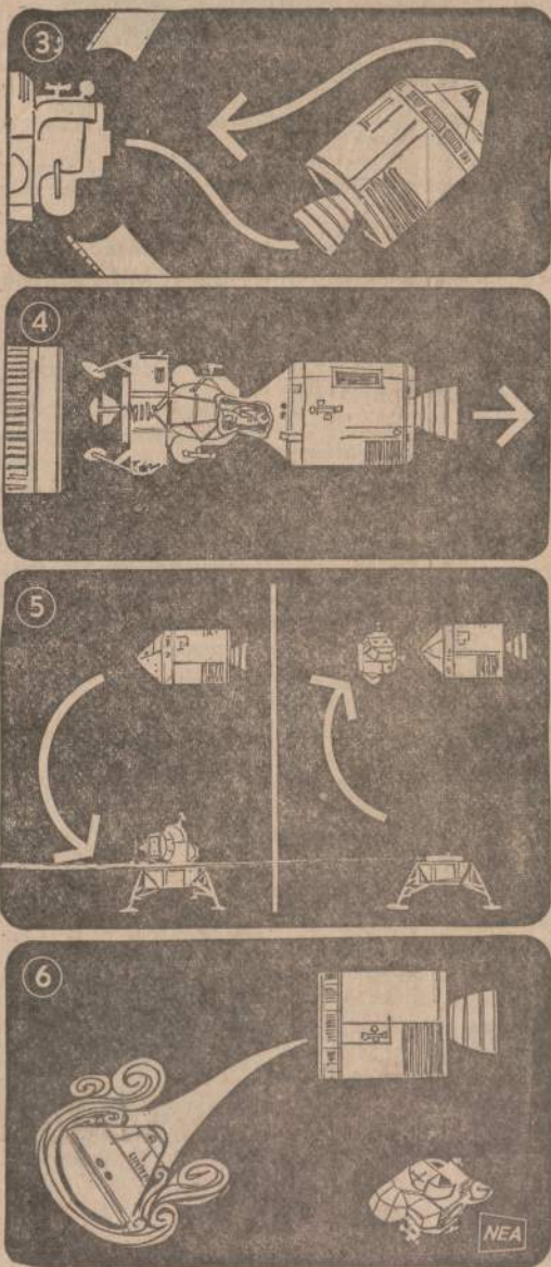
Trečių numerio pažymėtas paveikslas parodo, kaip Apollo 9 atsiskirs, o ketvirtu numeriu pažymėtas parodo, kaip didžioji Apollo 9 dalis vėl paims Lunar Module ir pakils į orbitą. Penktu numeriu pažymėtas paveikslas parodo, kaip Lunar Module atsiskirs nuo Apollo 9-ojo, paskraijos kokių šimto mylių atstumu, o vėliau vėl susijungs su Apollo 9. Tada du astronautai iš Lunar Module vėl perlips į Apollo 9. Šeštu numeriu pažymėtas paveikslas parodo, kaip astronautai paliks Apollo 9 lūktą, o pats erdvėlaivis leis į žemę.
