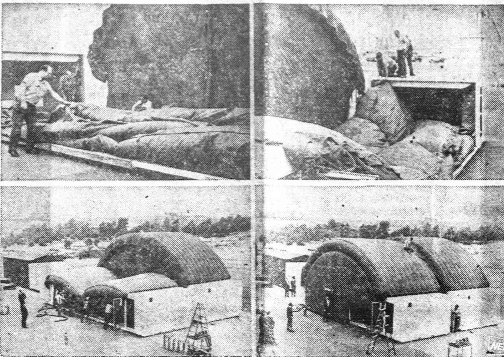
Amerikos aviacija jau pradėjo naudoti pripučiatus, didžiulius maišus barakams statyti. Tokie pastatai lengvai išardomi ir išvežami helikopteriais. Nuotraukose parodoma, kaip keli vyrai per trumpą laiką pastato nemažą baraką.
