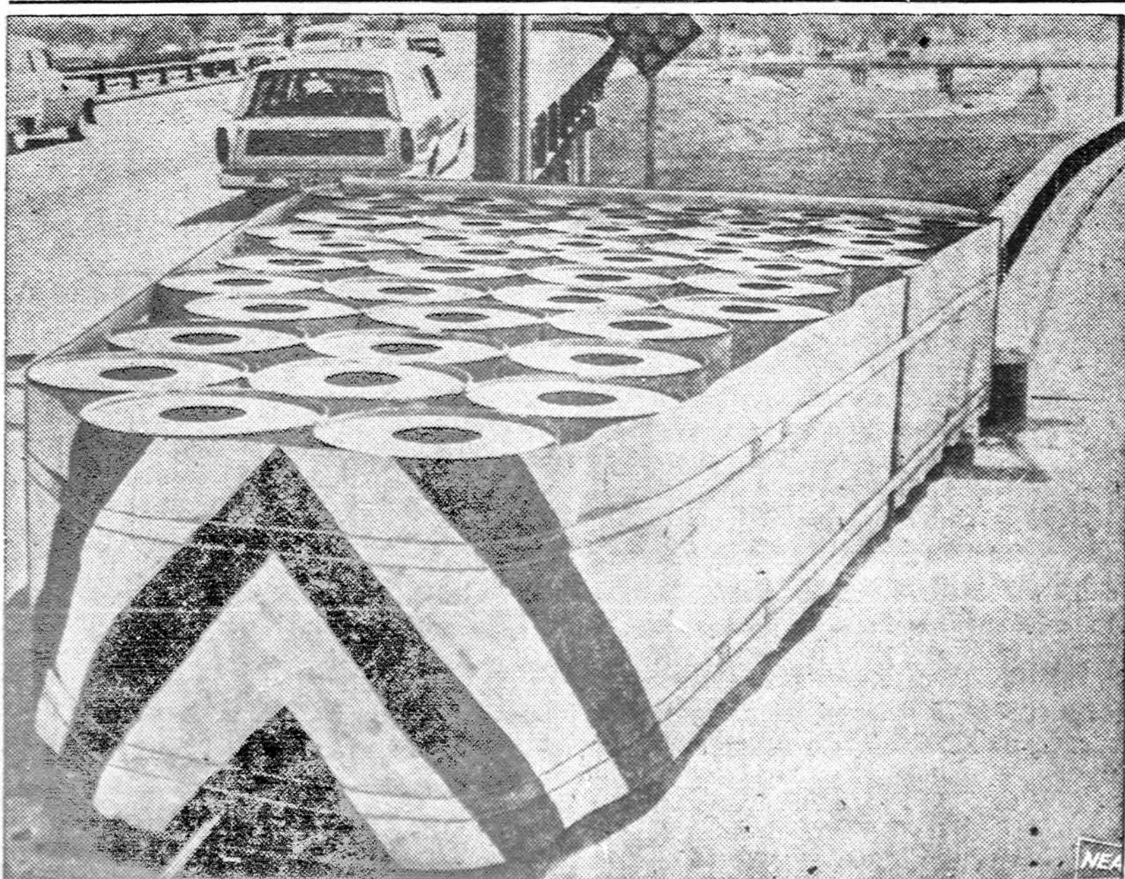
Šiame Houstono dviejų kelių susikryžavime anksčiau žūdavo daug žmonių. Dabar, vietoje cementinės užvaros pastatius šią 55 tuščių statinį buferį, dar neužsimušė nė vienas automobilistas.
