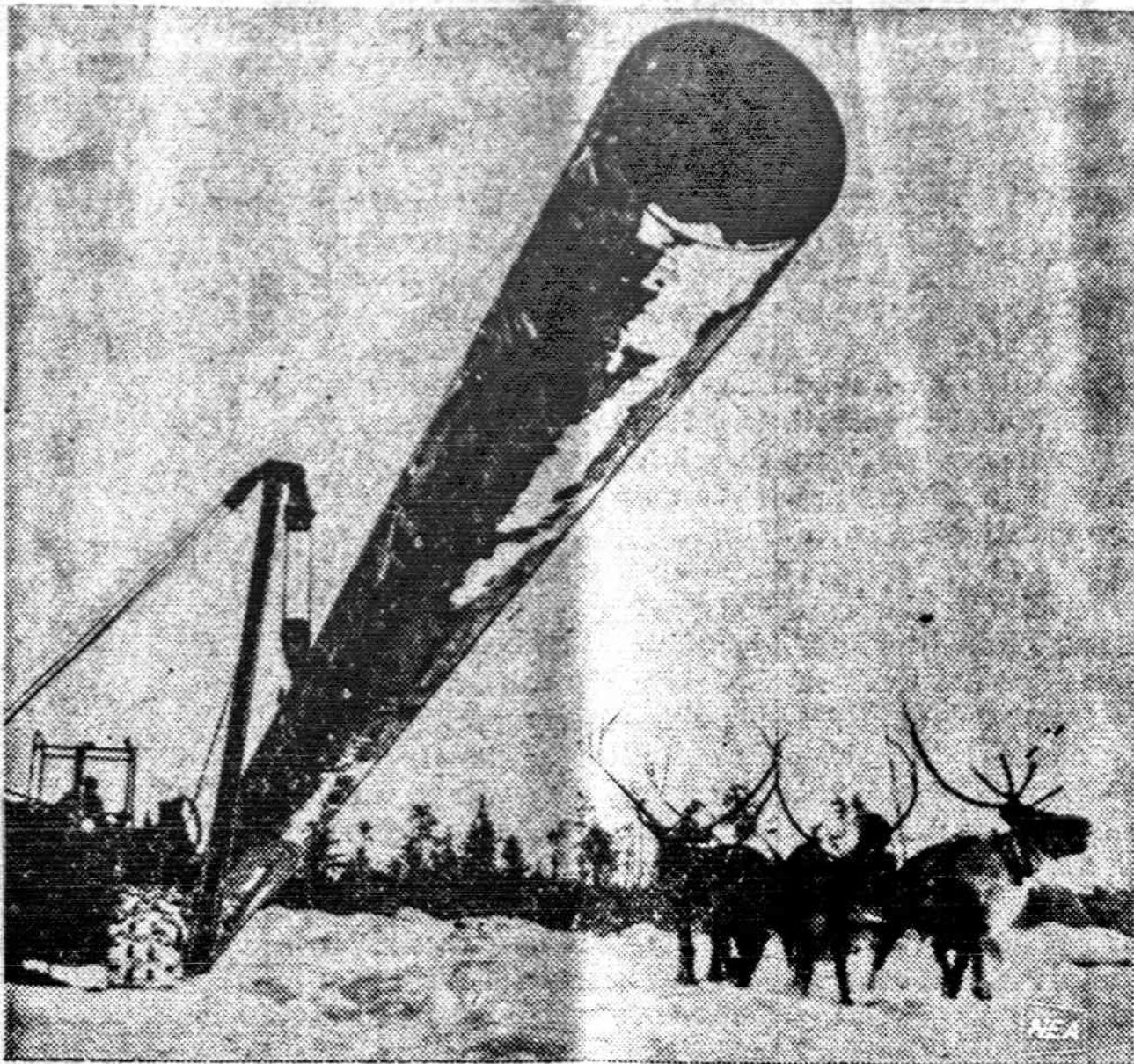
Sov. Sąjunga stengiasi išnaudoti Sibire esančius gamtos turtus. Tiesiamos vamzdžių linijos natūraliems dujoms. Šaltame ore tenka naudoti visokias susisiekimo priemones: traktorius ir brėdžius.
