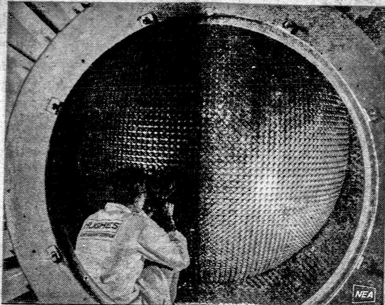
Į padidintą musės akį panašus paviršius iš tiesų yra naujo, pagerinto radaro „akis“, kuri bus naudojama Amerikos padangų gynybai. Ją montuoja Hughes įmonės inžinierius.
