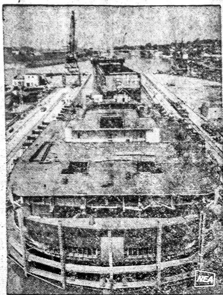
Lorain, Ohio statomas didžiausias Didžiųjų Ežerų laivas. Tai bus U. S. Steel bendrovės geležies rūdos vežiotas, jo ilgis 858 pėdos.
