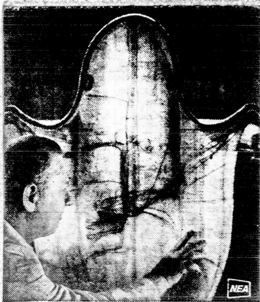
Iš pirmo žvilgsnio gali atrodyti, kad čia mokslininkas tyrinėja per- šviesto žuvies nervus. Tikrovė yra visai kitokia. Šis inžinierius fi- krina sprausminio lėktuvo sparnus šildomas vielas. Jei vielos ne- bus tiksliai suldytos, tai ant lėktuvo sparnų pradės formuotis ledo sluoksnis.
