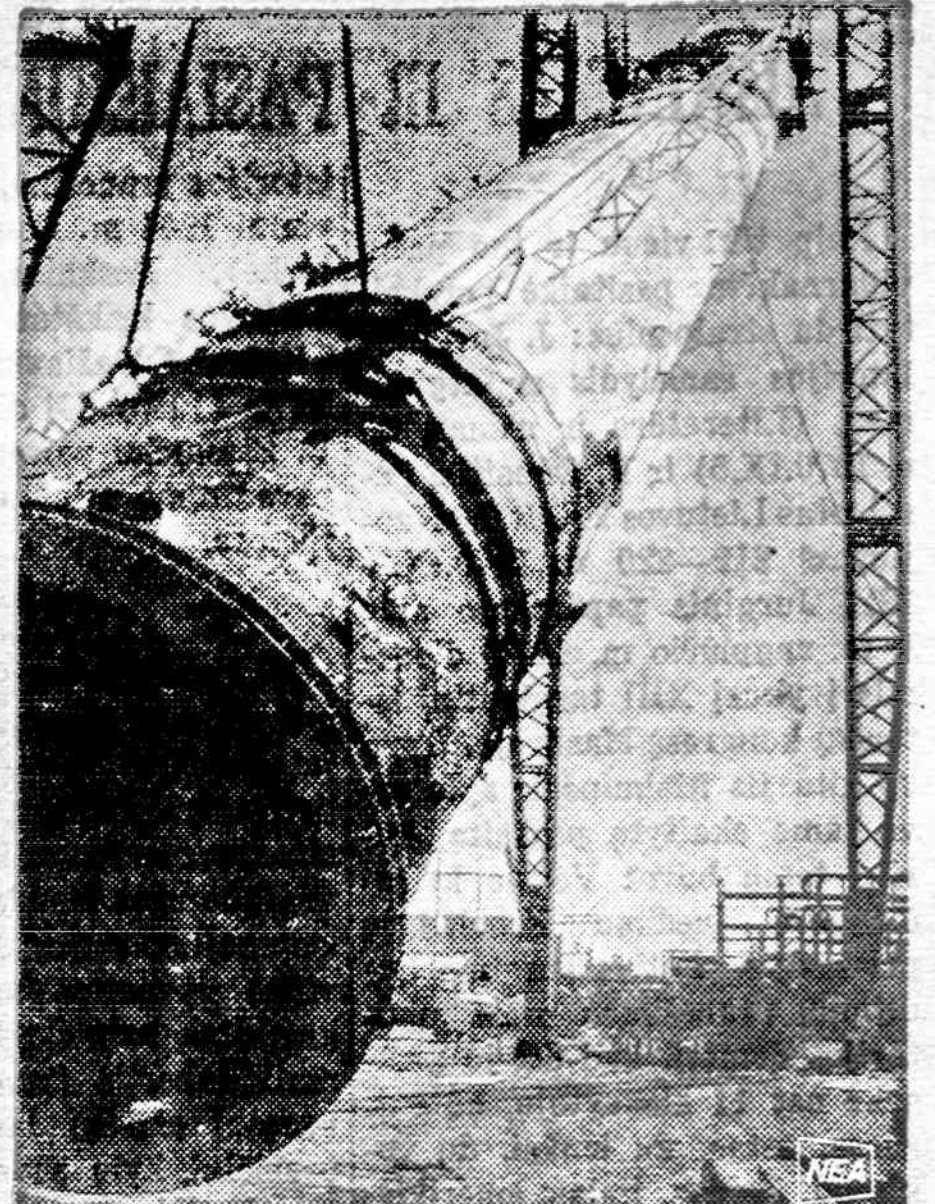
Tai 206 pėdų ilgio propylene dujomis leisti vamzdis. Vamzdis padarytas iš beveik dviejų colių storio plieno lakštų. Teko lydinai 11,000 pėdų, kad suvirintus tokį vamzdį. Vėliau teko padaryti 1,750 rentgeno nuotraukų, kad patikrintų, ar sulydinimas yra be plyšių. Teko pastatyti specialius vagonus, kad šį vamzdį iš Luisianos, Shreveport miestelio galėtų nugabenti į Texas valstiją, Odesos miestelį.
