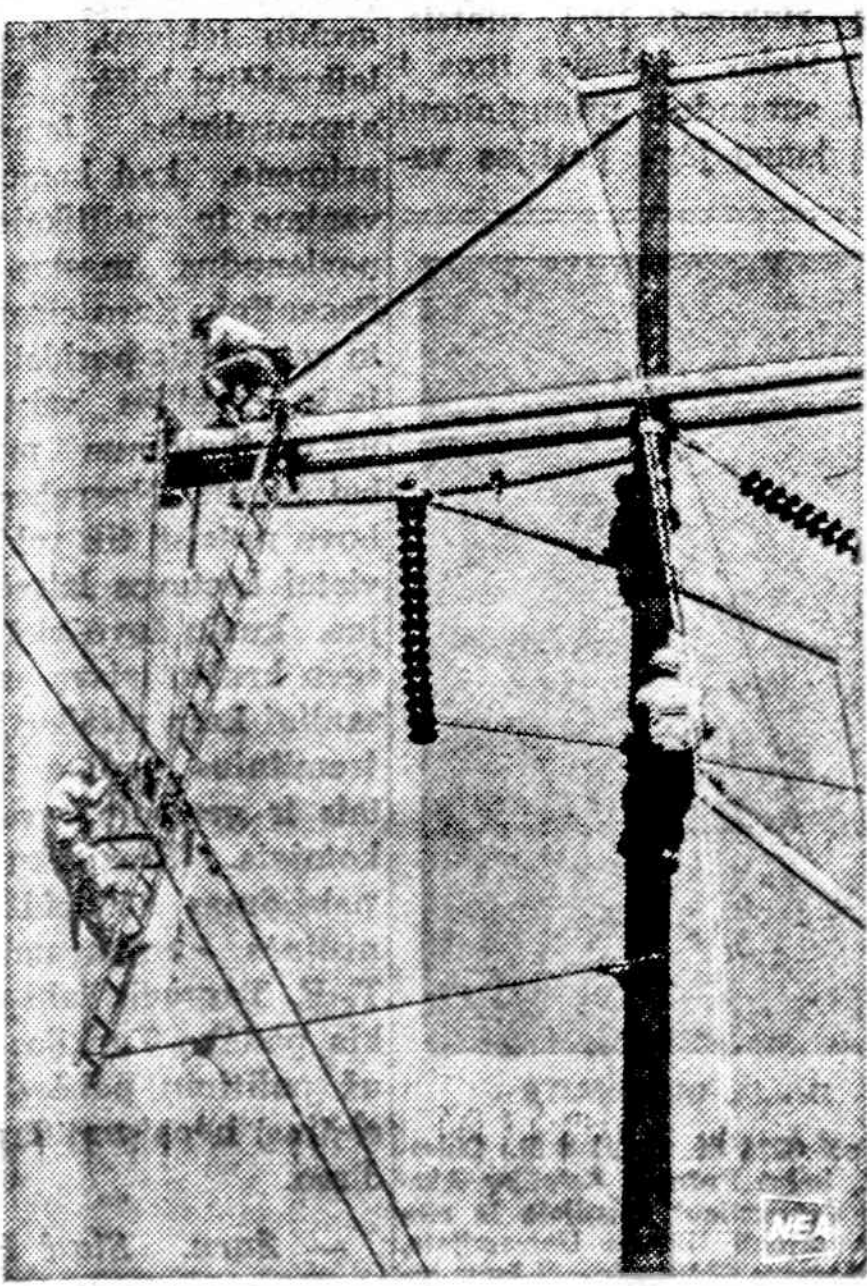
Stiklinio pluošto ir plastmasės mišinys vis plačiau naudojamas. Pa- veiksle matomam elektros stulpui visos dalys gamintos iš naujo mi- šinio, net ir darbininkų kopėčios.
