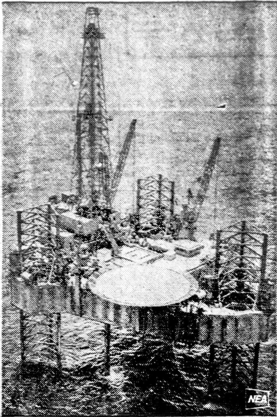
Meksikos įlankoje statoma nauja platforma naftos šaltinių ieškojimui jūros dugne. Ant platformos stovi gyvenamieji namai ir yra apskrita vieta helikopteriams nusileisti.
