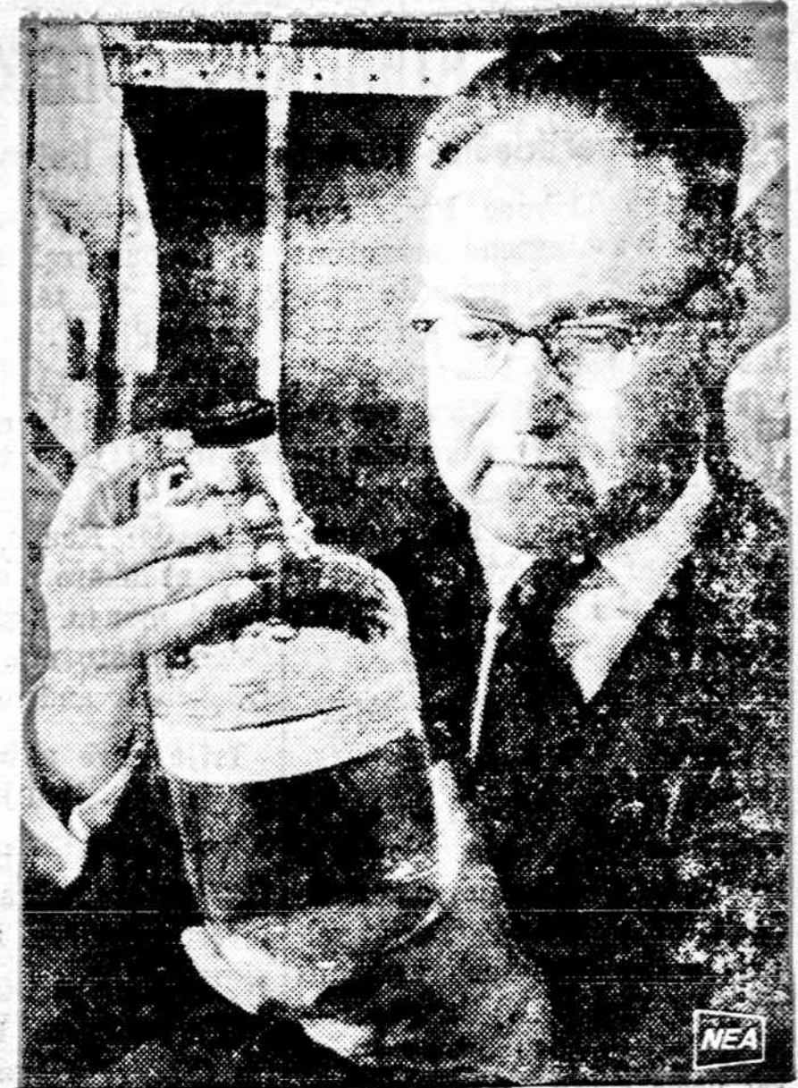
Izraelio Waitzmano Institute laikomas labai senas vanduo, rastas Negevo dykumos olose. Išmatavus vandens amžių, manoma, kad jis turi 20,000 metų.
