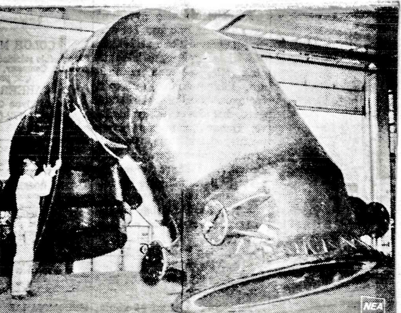
Iš stiklinio pluošto pagaminta "alkūnė" bus įteista Texas medžio apdirbimo įmonei. Vamzdis yra 5 pėdų, šešių colių skersmens ir sveria 4000 svarų. Jis nerūdijia, yra stiprus bei atsparus.
