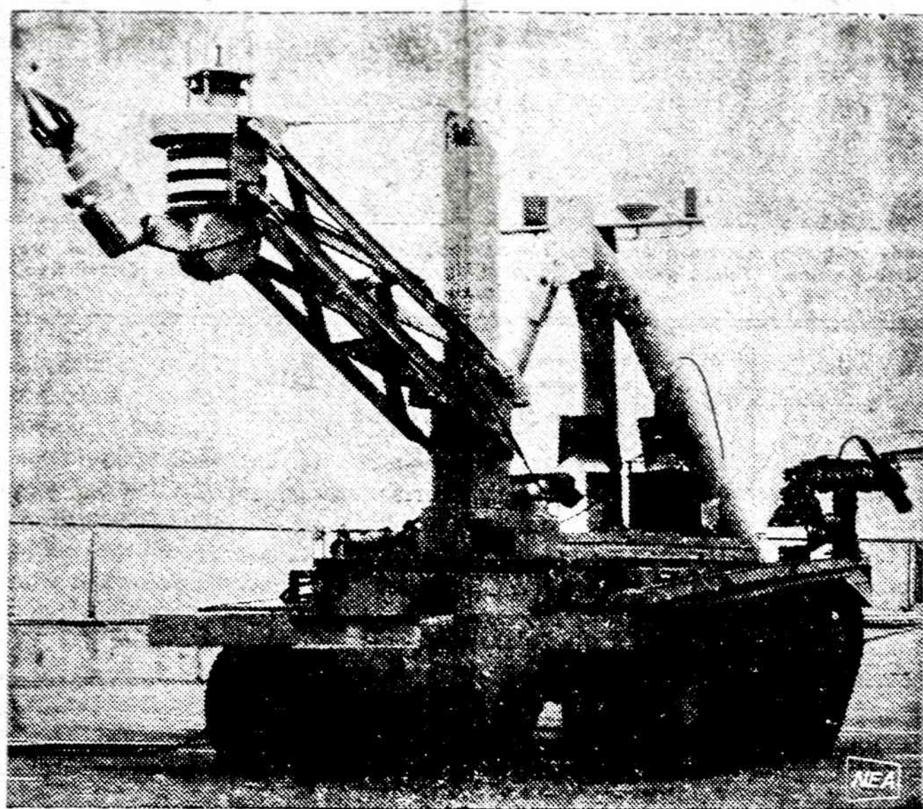
Moderni jūrų baidyklė yra šis RUM (remote underwater manipulator) tankas, kuris važinėja jūros dugnu netoli La Jolla, Kalifornijoje. Šis robotas gali pakelti daiktus dugne ir juos nufotografuoti.
