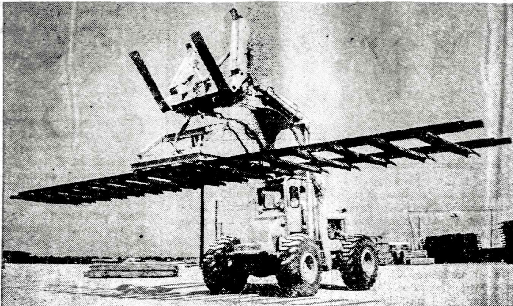
Amerikijoje pradėti gaminti geležinkelio bėgiai kartu su plieno pabėgiais. Jie naudojami prekybos stotyse ir šalutinėse linijose. Šitokias linijas nutiesti su naujais bėgiais yra, palyginti, greitas darbas, ypač kada naudojamos didelės masinės.
