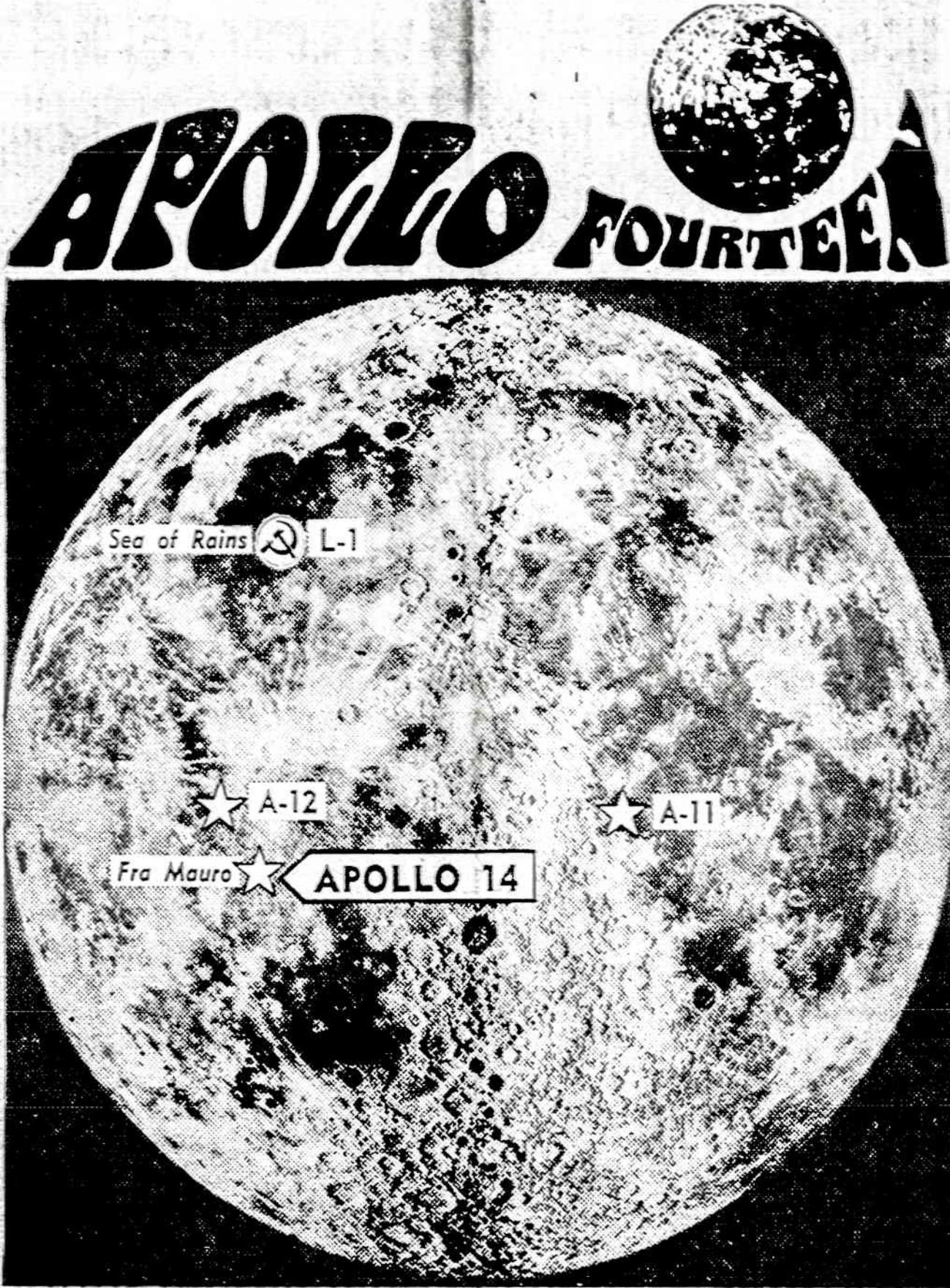
Piešinys parodytos vietos, kur jau buvo nusileidę Amerikos astronautai: A-11 ir A-12. Apollo 14 nusileis Fra Mauro vietovėje. Viršuje parodyta vieta, kur buvo nušautas sovietų Lunochod-1.
