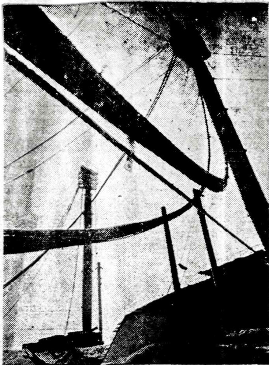
Olimpiniai žaidimai 1972 metais dar toli, tačiau pasirošimai Muenchene, V. Vokietijoje, vyksta pilnu tempu. Šie pilno lynai laikys didelį audeklinį stogą.
