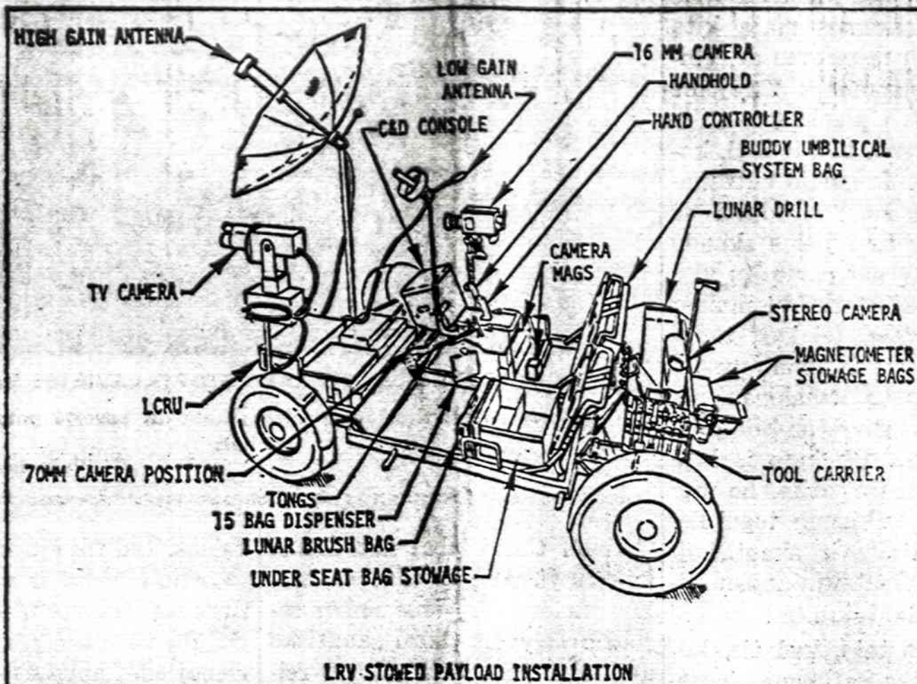
Šis brėžinys parodo įrengimus amerikiečių mėnulio automobilio, kuris bus nuvežtas į mėnulio liepos mėnesį.
