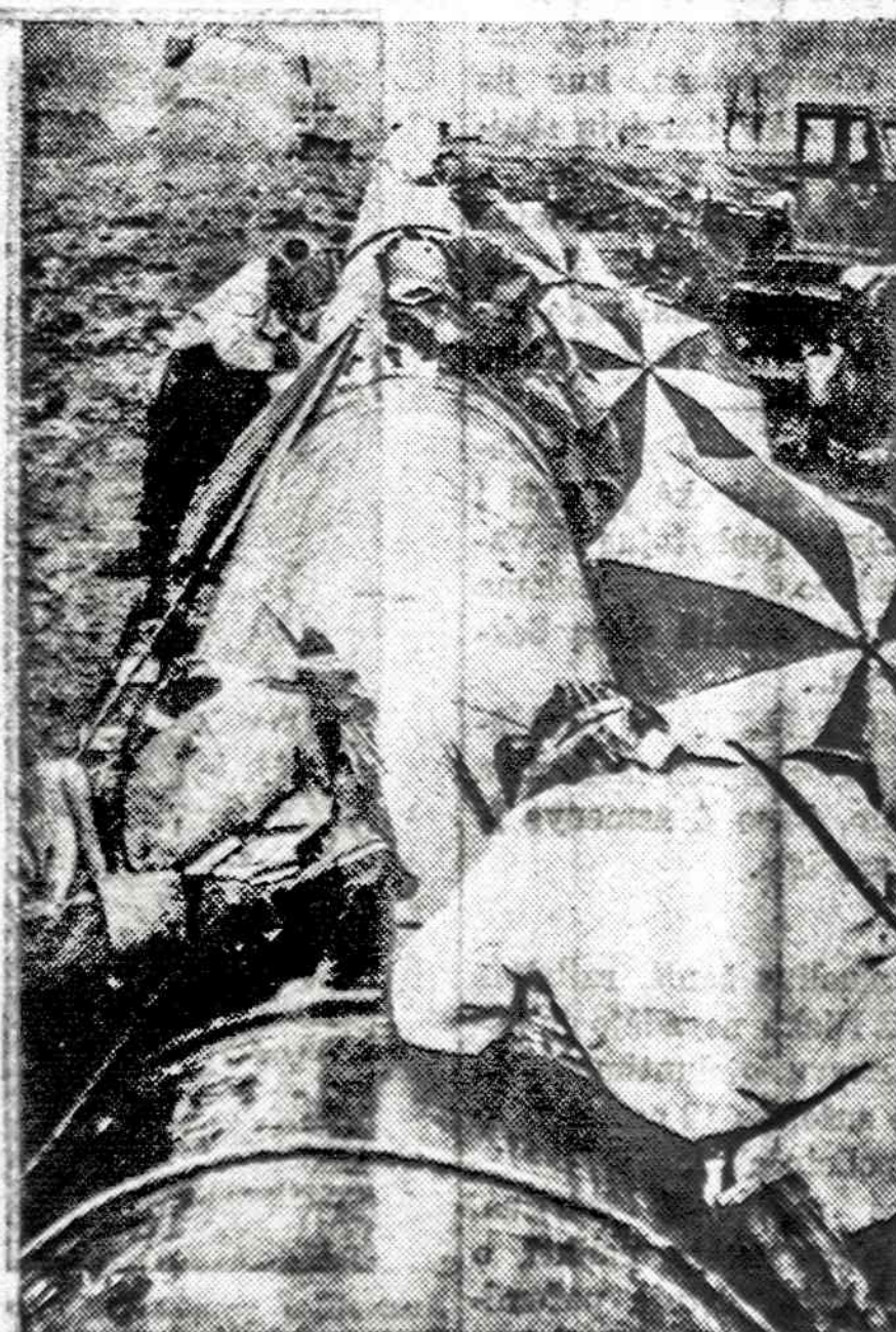
Čekoslovakijoje tiesiama naftos vamzdynų linija. Darbas nesustoja ir lygiagrečiai. Darbininkai turi netoliese pasidėti Hetsargio, po kuriais tęsiasi darbas.
