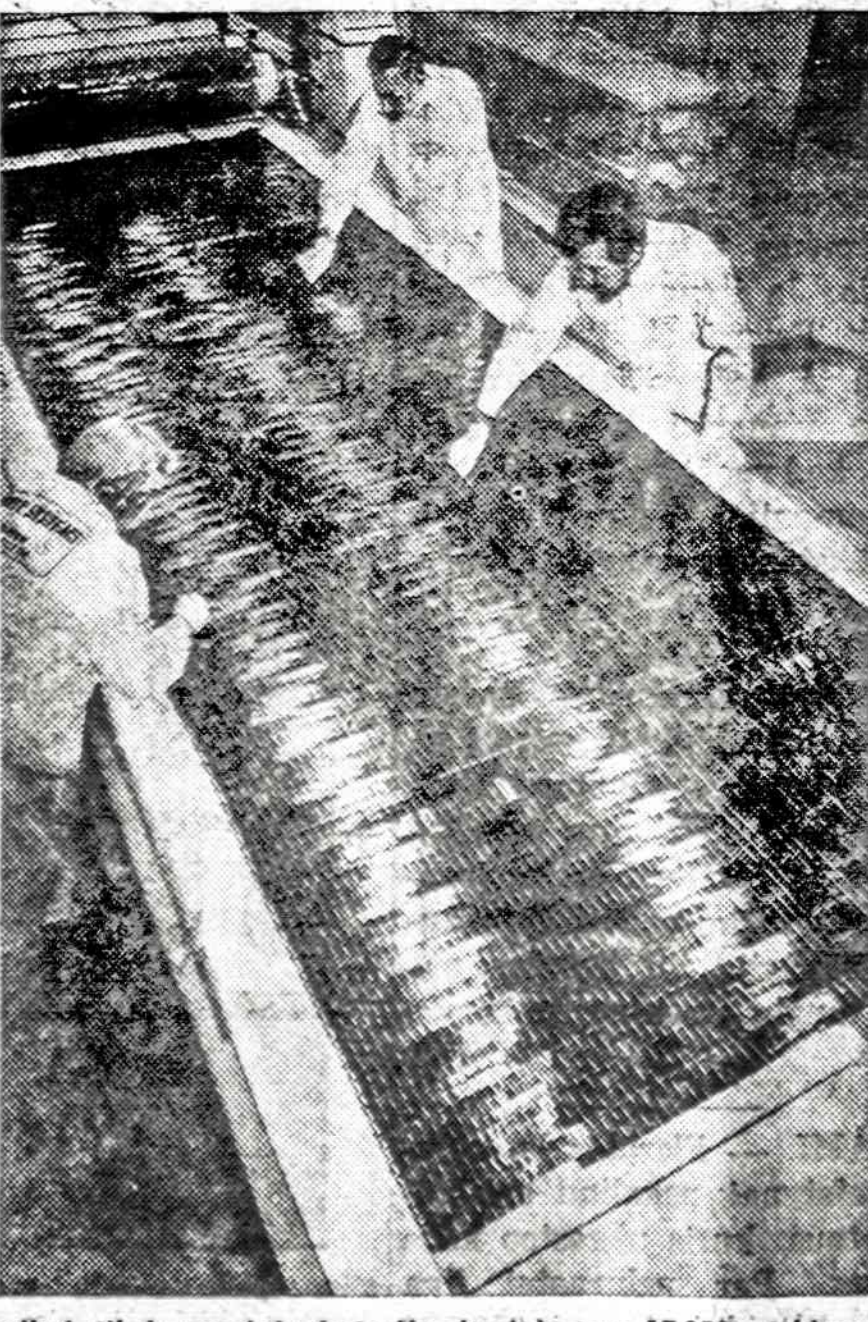
Technikai tikrina erdvės bateriją, kurioje yra 17,250 atskirų celių. Erdvėlaiviai tą bateriją iškelti suvyniota, tačiau ji išsitiesia erdvėje ir saulės spindulių palietusios celės gamina elektros energiją, net 1,500 vatų pajėgumo. Suvyniota baterija tampa tik 10 celių cilindru, o ištiesa sudaro 32 pėdų "paklodę".
