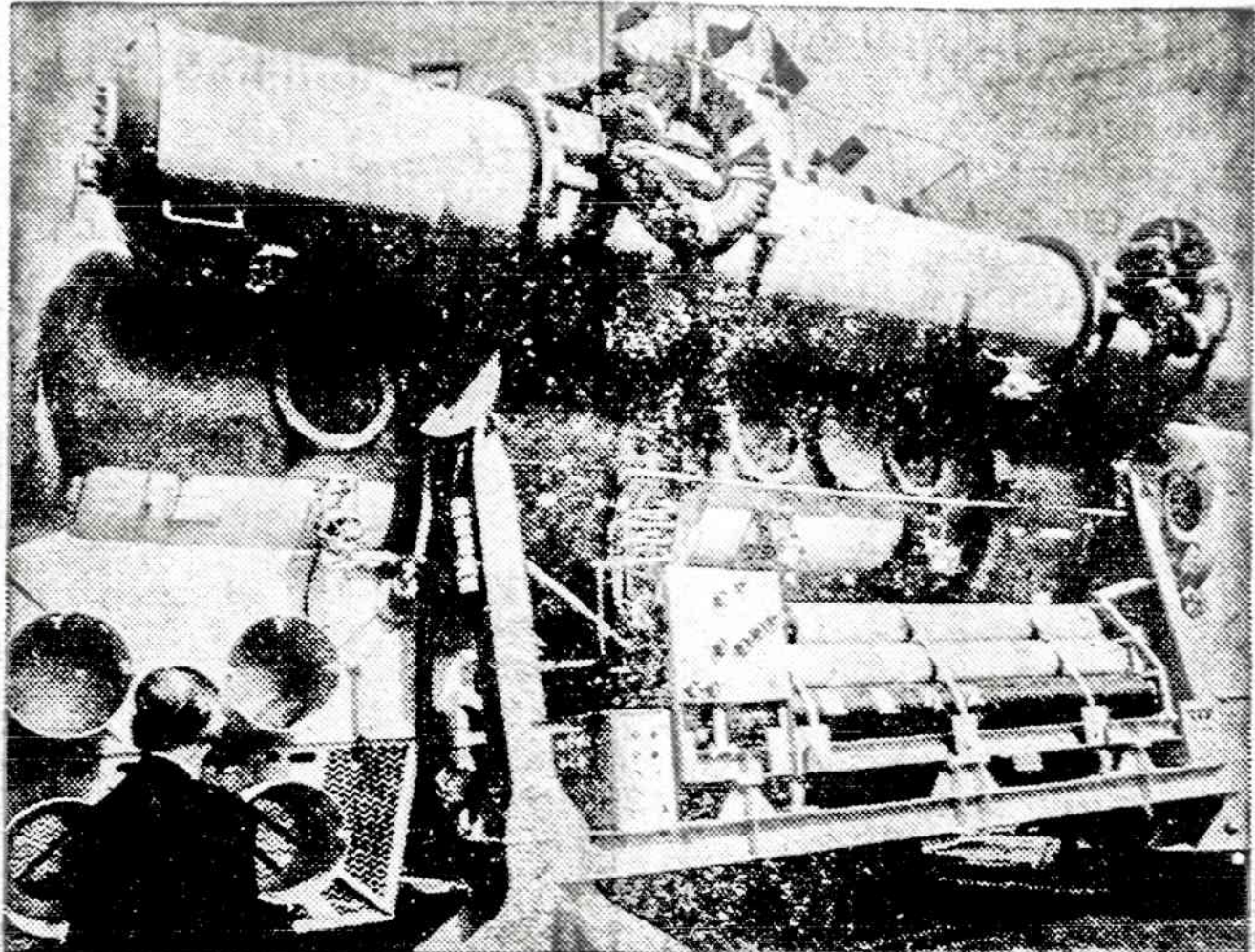
Japonijoje pastatyta jūros dugnui tirti laboratorija turi 33 pėdas ilgio, 13 pėdų pločio ir 21 pėdą aukščio. Viduryje yra darbo ir poilsio patalpos keturiems žmonėms.
