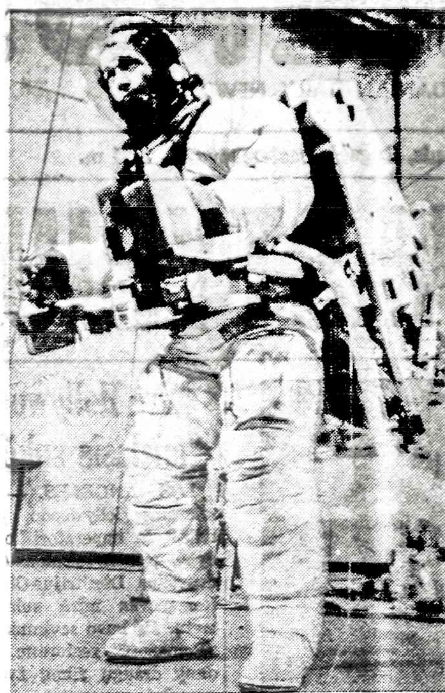
Astronautų drabužiai vis tobulinami, pritaikant juos ateities kelionių užduotims. Šiame paveikslė parodomas astronautų nešiojamas aparatas, kuris susideda iš sprausminių motorėlių, kurie nešioja astronautus po dideles erdves stotis. Rankomis vairuojamos motorinės kuprinės gali skristi 30 minučių su visu astronautu. Paskui vėl jas reikia pakrauti.
