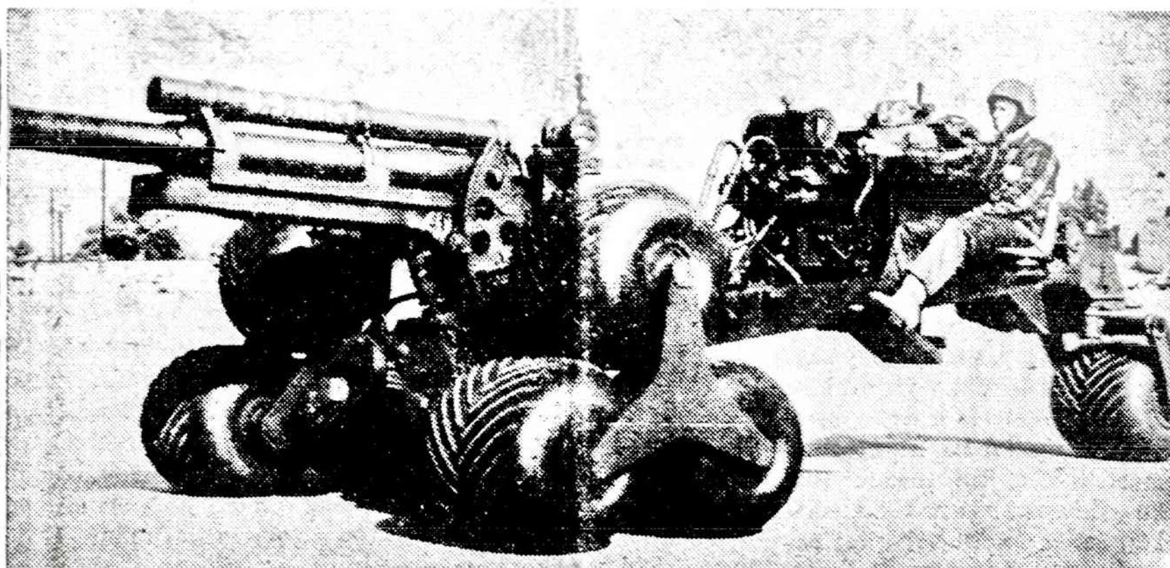
Nauja Amerikos 105 mm. patranka yra labai judri. Ją pagamino Lockheed Aircraft bendrovė. Patranka gali važiuoti per gilų dumblą, pelkęs ir nelygias, akmenuotas vietas.
