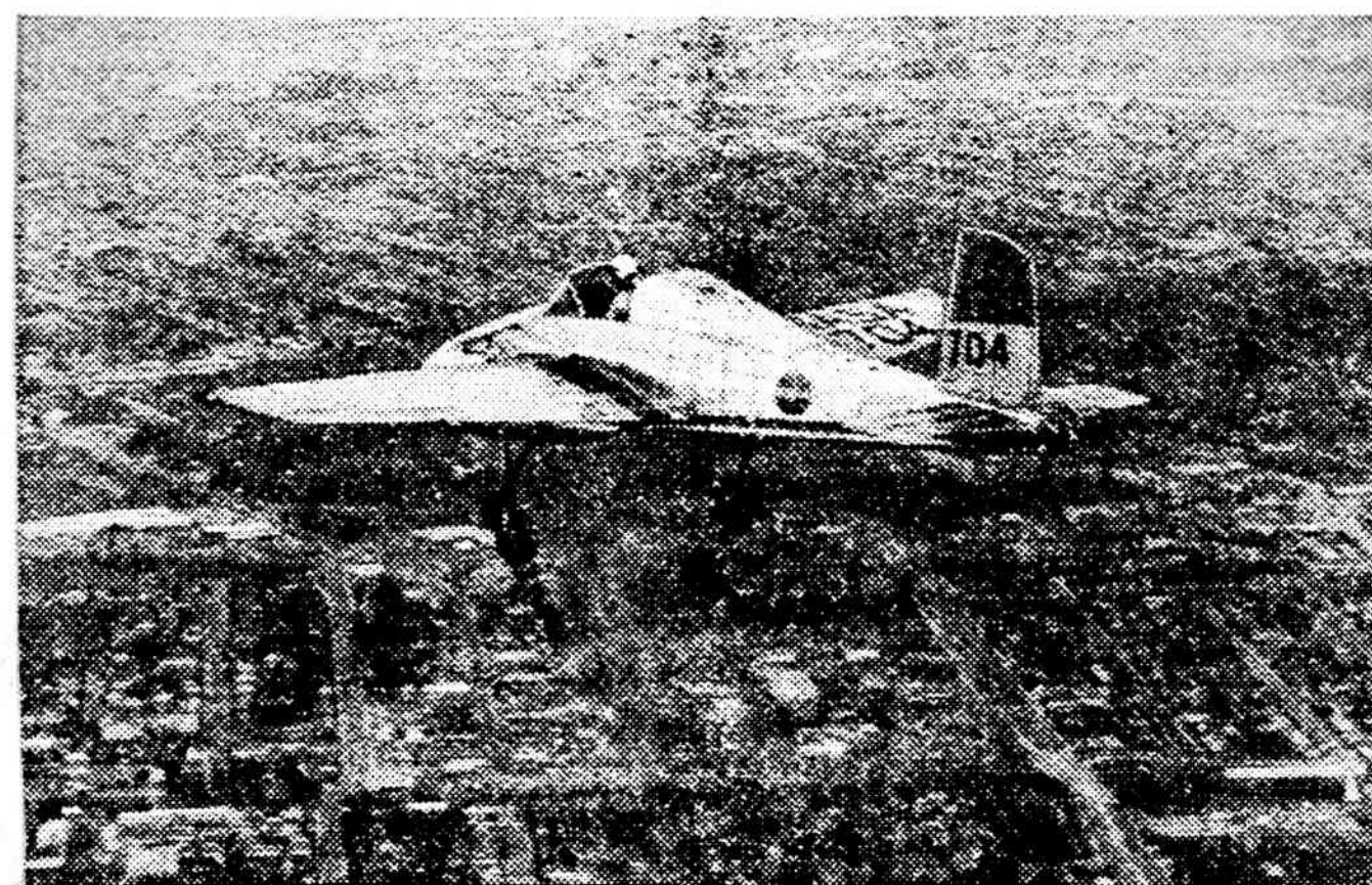
Nasa bandymų centre, Mountain View, Calif., bandomas naujas lėktuvas, kuris pakyla stačiai į viršų be įsibėgėjimo ir taip pat nutopia ant žemės. Lėktuvas X-14B turi kompiuterių įrengimus, kurie padeda apskaičiuoti skridimo charakteristikas kitų panašių lėktuvų — VTOL (vertical take-off and landing), kurių bandymų ar konstrukcijos stadijoje yra keli modeliai.
