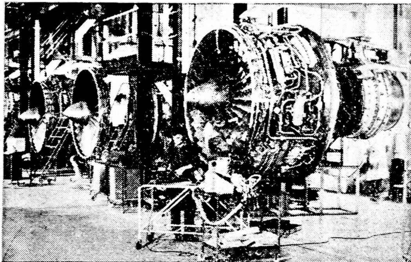
Britanijos Rolls-Royce įmonėje Derby yra statomi motorai Amerikos Lockheed bendrovės statomam Tristar lėktuvui. Motorai turi 42,000 svarų sprausminę jėgą.
