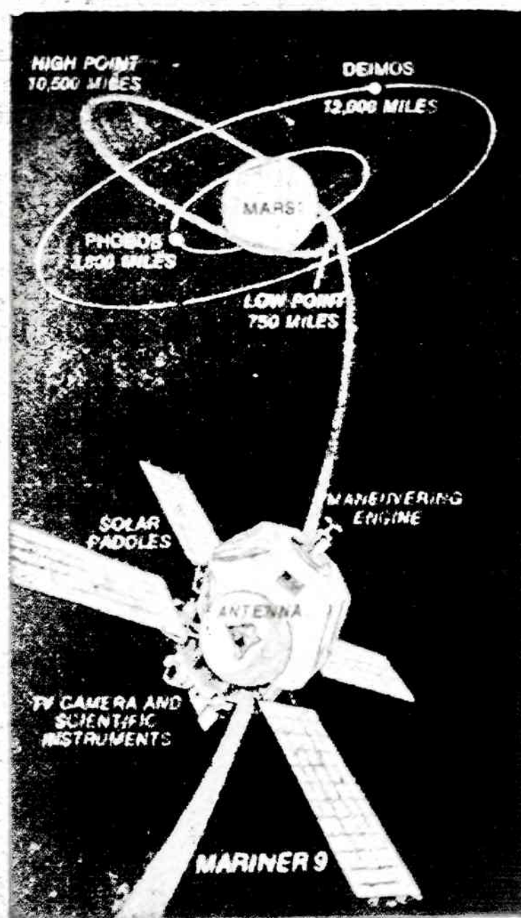
Šiame piešinyje matomas Mariner 9 erdvėlaivis pradėjo fotografuoti Marsą ir du jo palydovus. Iš ankstyvesnių fotografijų pastebima, kad Marso mėnuliui Phobos ir Deimos nėra visiškai apskriti, bet panašūs į kiaušinių. Phobos esąs 21 mylios ilgumo ir 18 mylių platumo.
