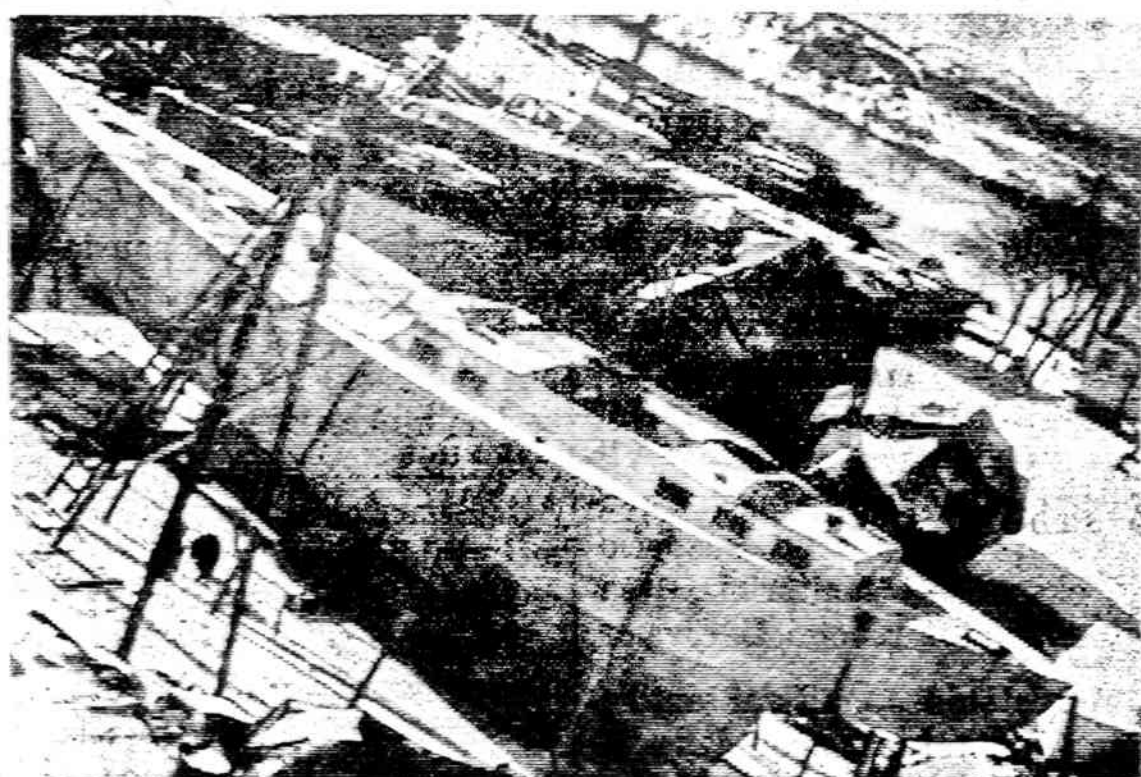
67 pėdų ilgio gelžbetoninės jachtos cementu apipiltas liemuo Gleason Marina laivų dokoje. Laiku įsidėjus langus ir kt. uždengimus, savininkas viduje ir per šią žiemą dirba prie vidaus įrengimų, nes vidų apšildo.
