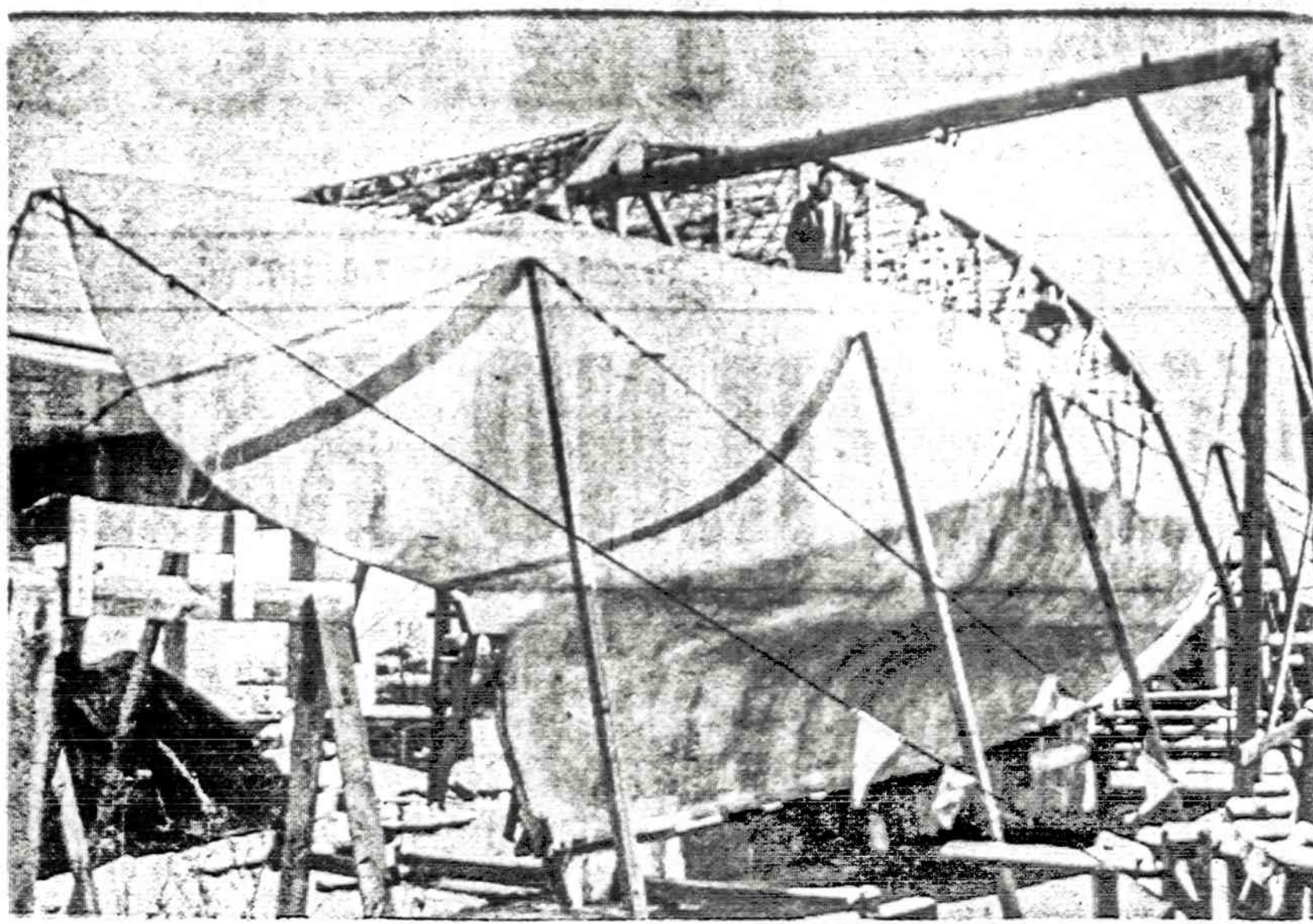
Gelžbetoninės burinės jachtos liemuo, žiūrint nuo žemės. Viršuje stovi laivo savininkas p. L. W., o kiek toliau jo sūnus George.
